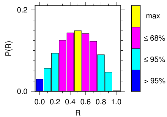
(d) shape ratio
