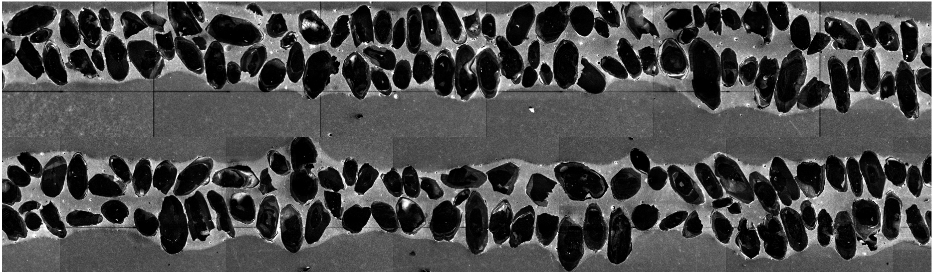
575 Granite (3013 Ma)
