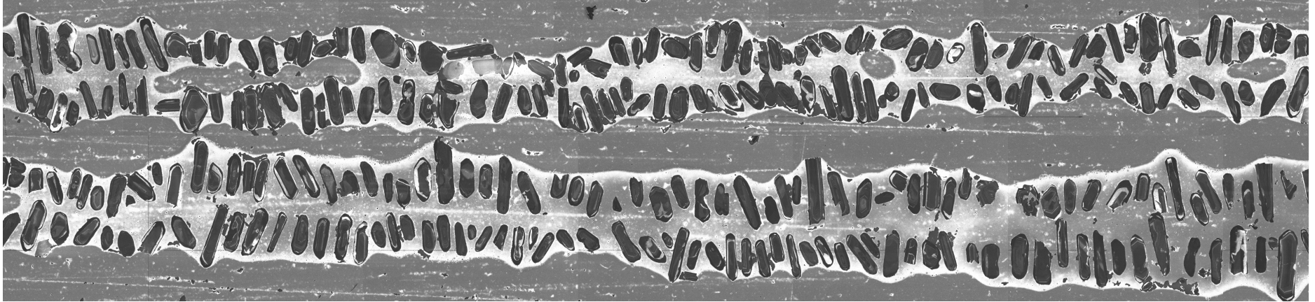
739 Psammite
