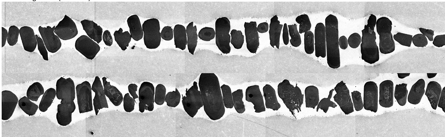
318 Pegmatite (2729 Ma)
