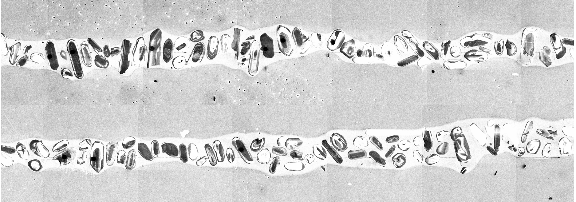
566 Tonalite (3018 Ma)
