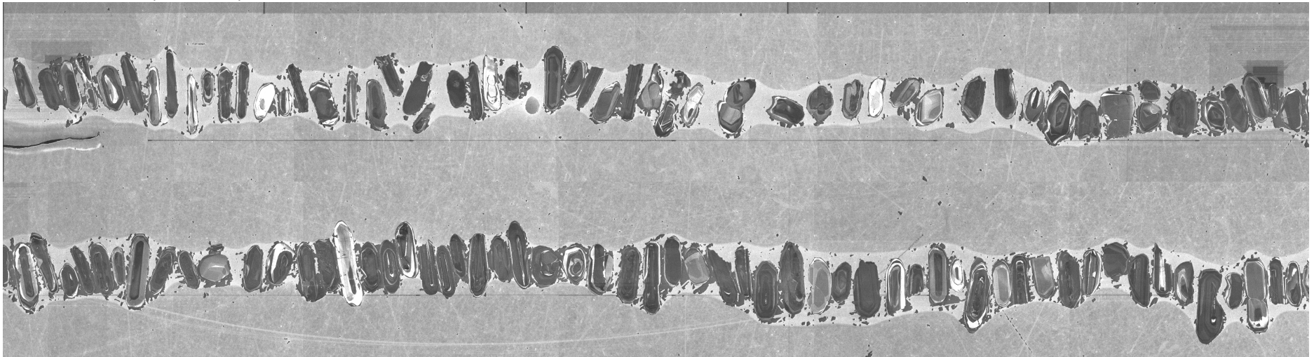
306 Tonalite (3019 Ma)
