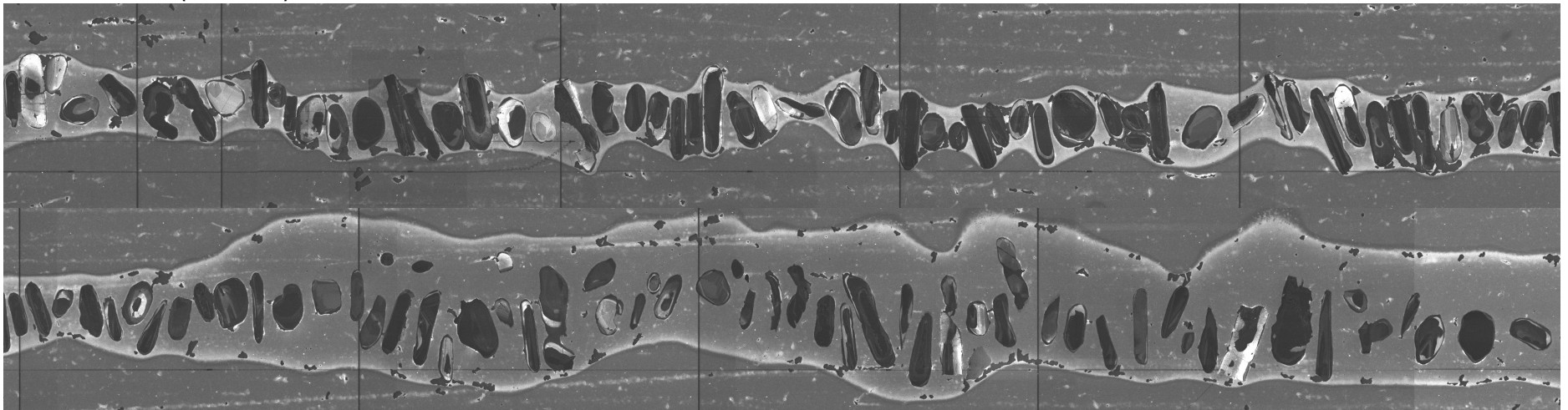
325 Tonalite (3002 Ma)
