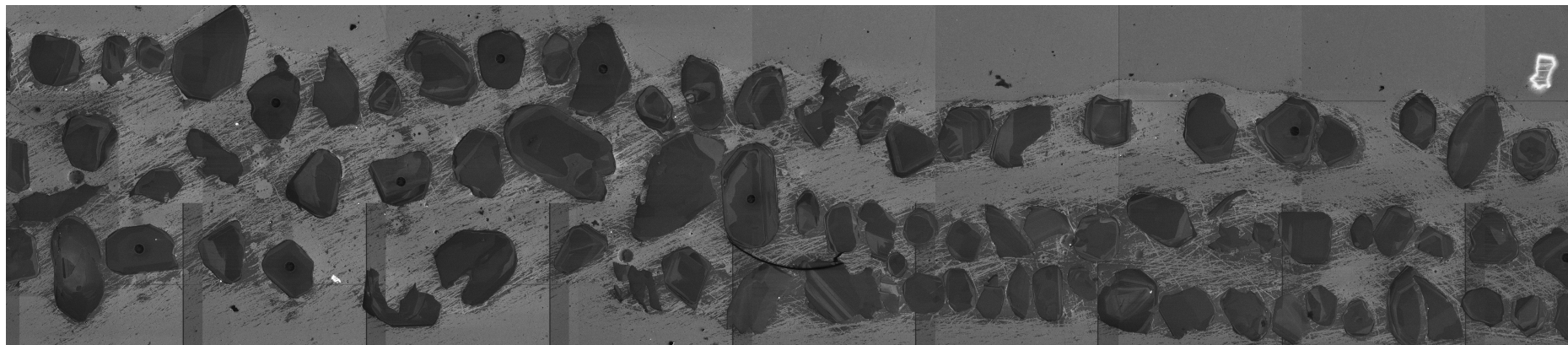
318 Pegmatite (2729 Ma)
