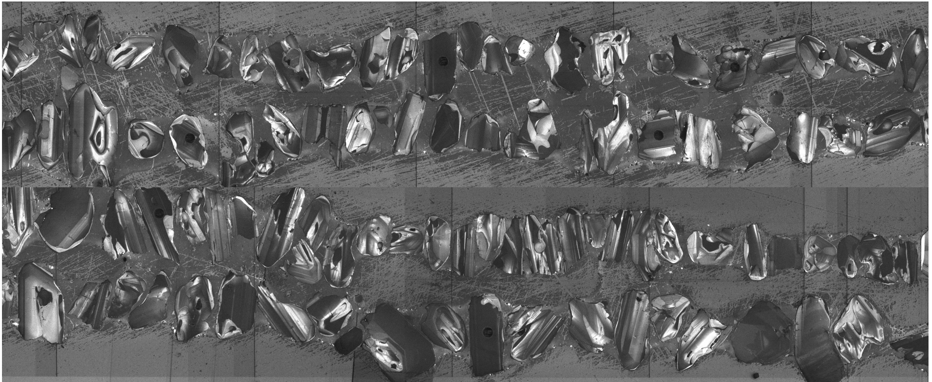
173 Leucogabbro (3007 Ma)
