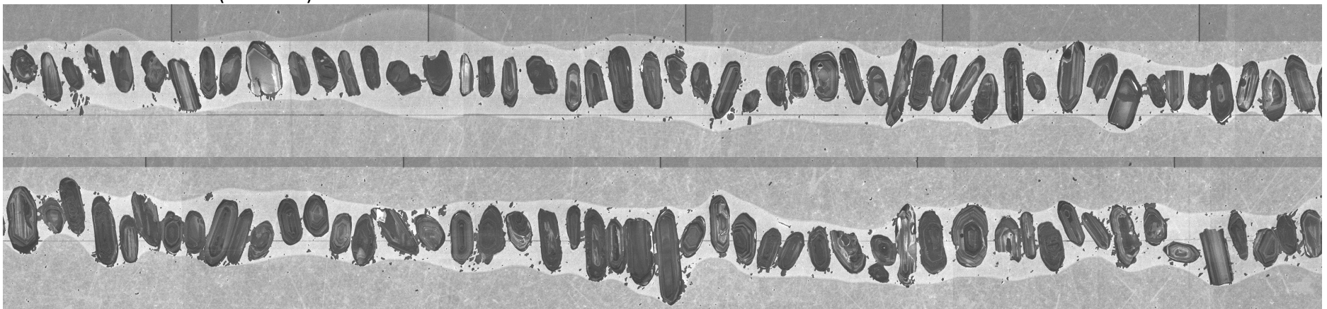
307 Diorite-tonalite (3011 Ma)
