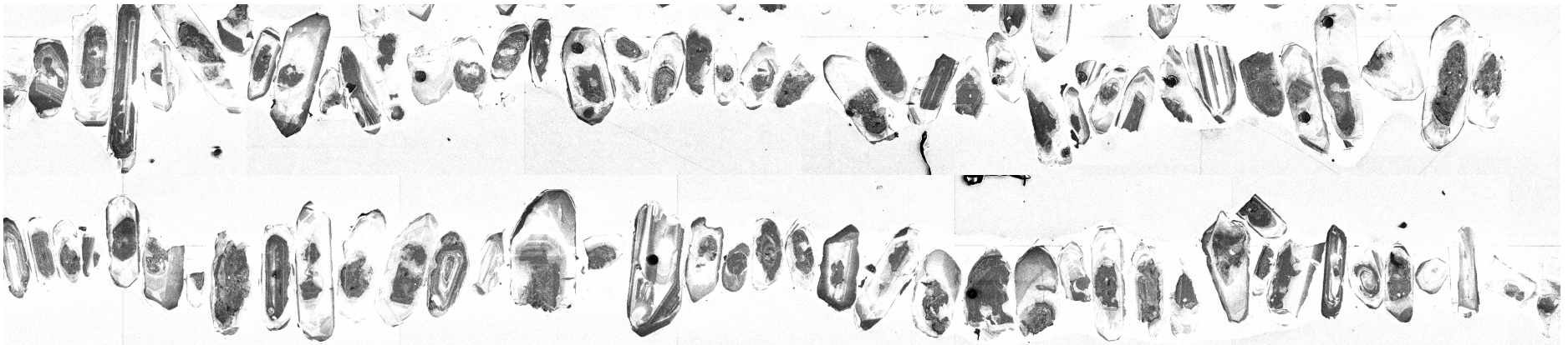
224 Granite (2986 Ma)
