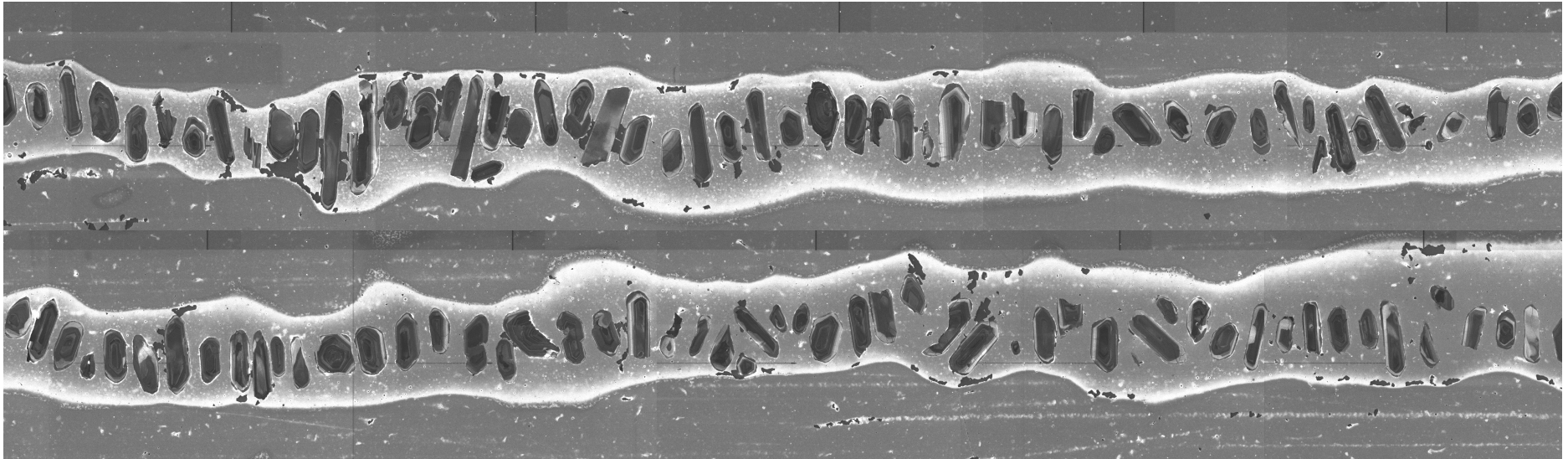
407 Tonalite (2994 Ma)
