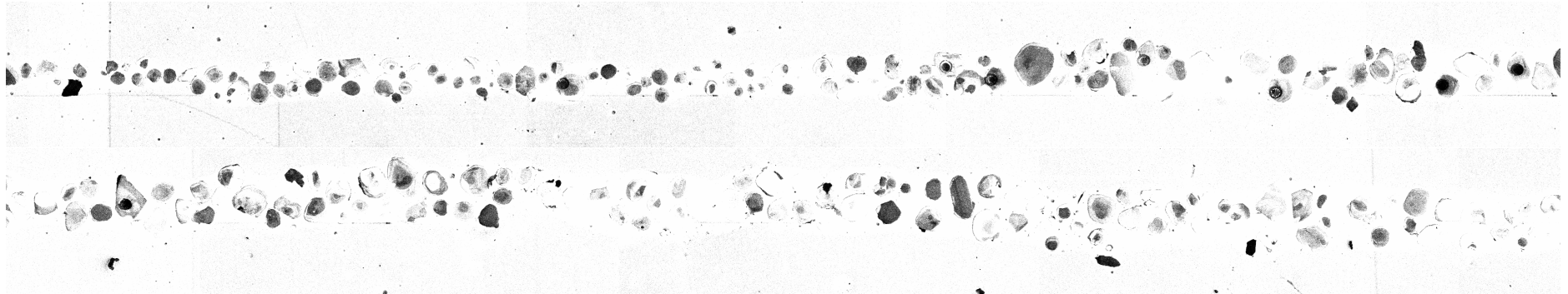
483 Paragneiss
