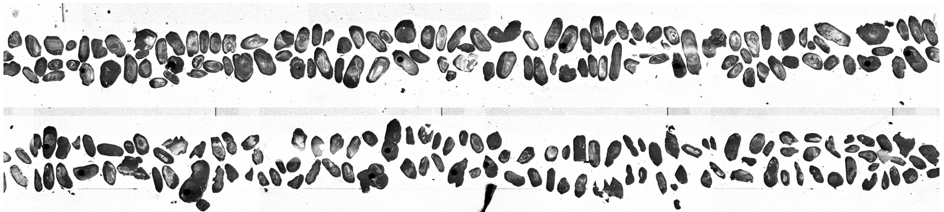
537 Paragneiss
