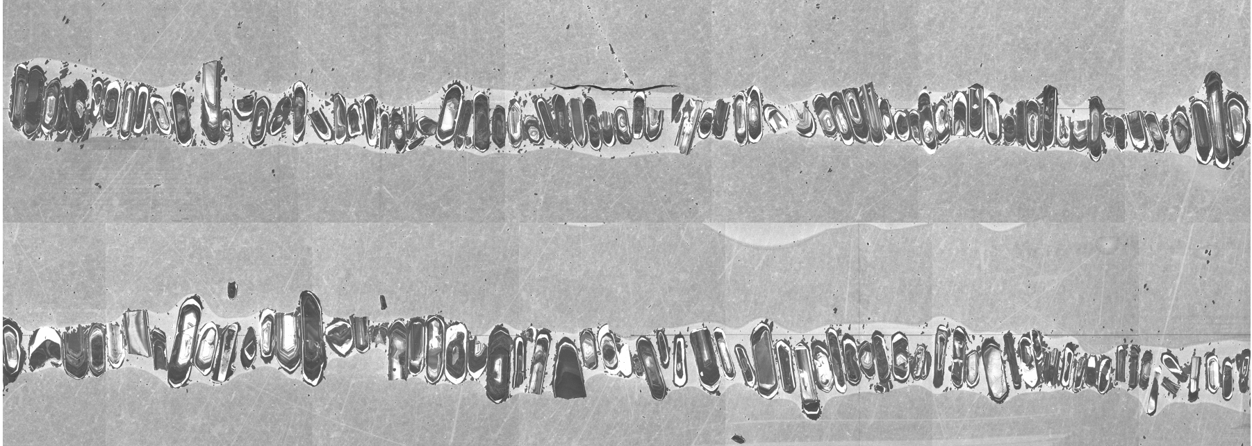
222 Trondhjemite (3240 Ma)
