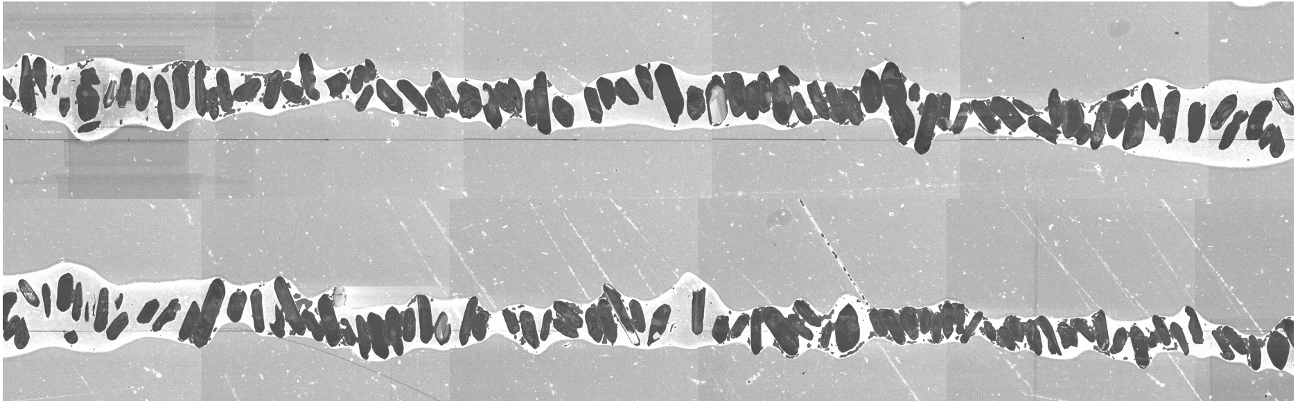
221 Granite (2977 Ma)
