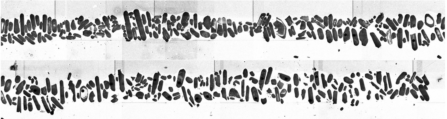
535 Paragneiss
