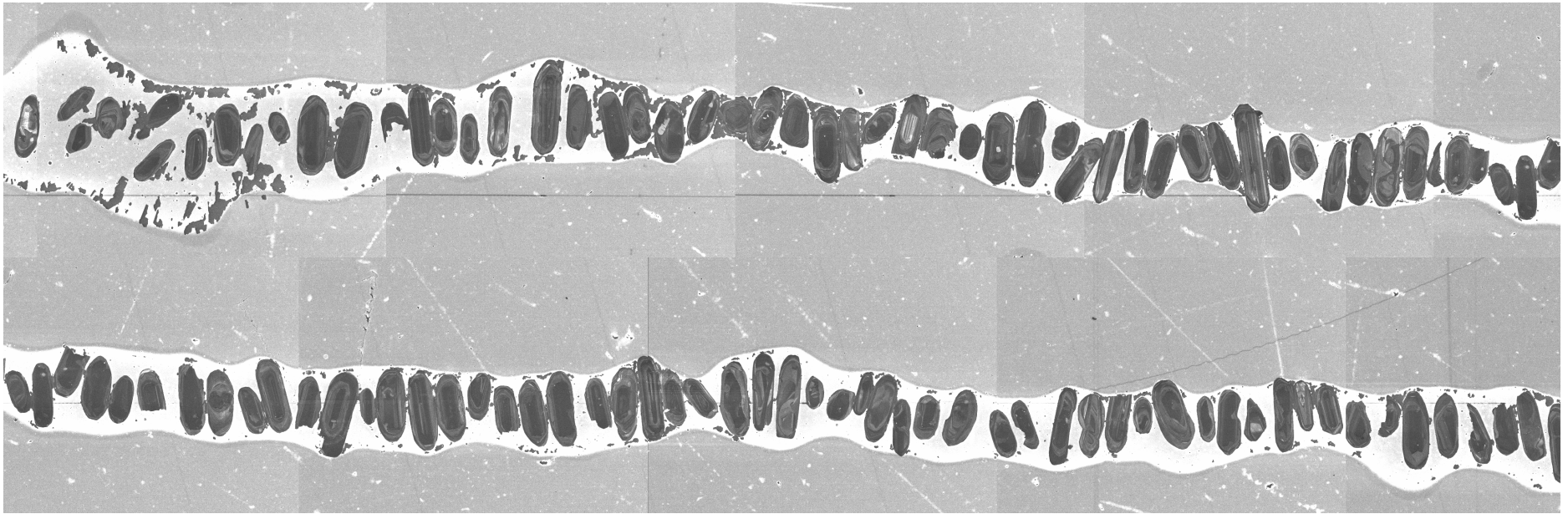
235 Tonalite (2992 Ma)
