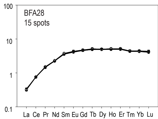
Clinopyroxene
