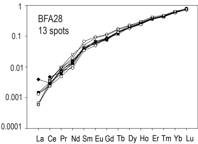
Orthopyroxene
