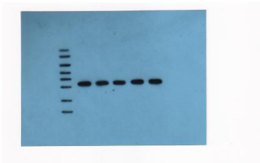
Fig 5B-1 FOSL1
