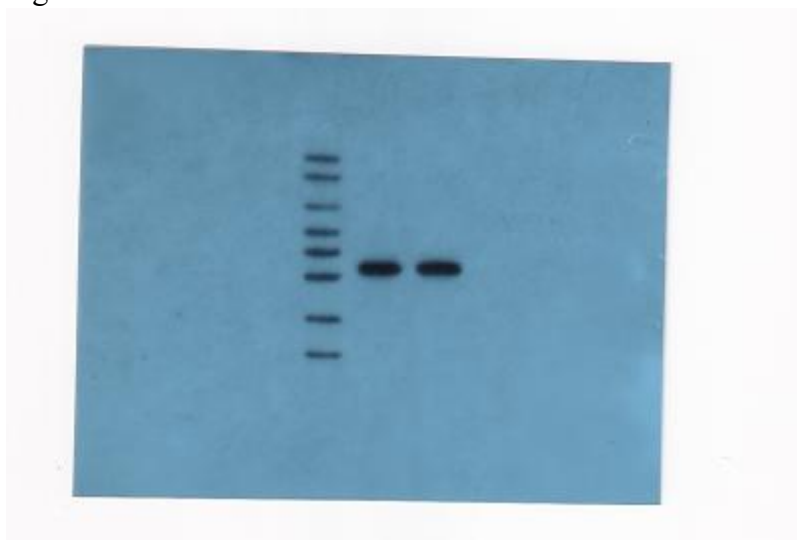
Fig 6C-1 VDR
