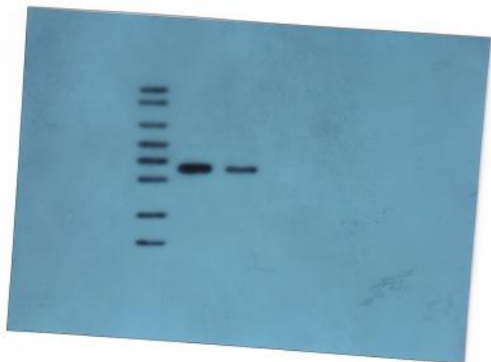
Fig 6F-2 VDR
