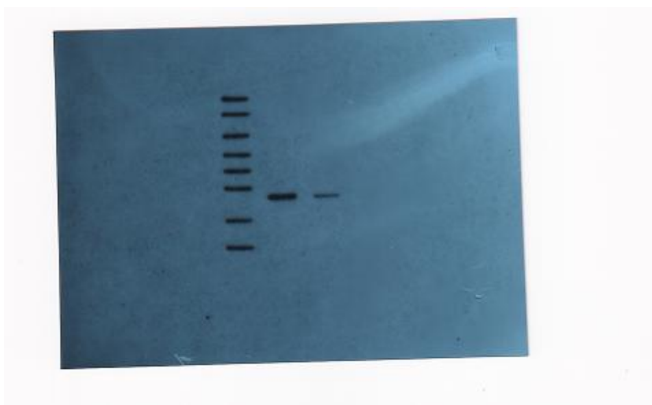
Fig 5B-1 FOSL1
