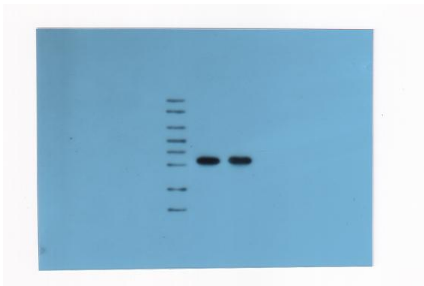
Fig 6F-1 FOSL1
