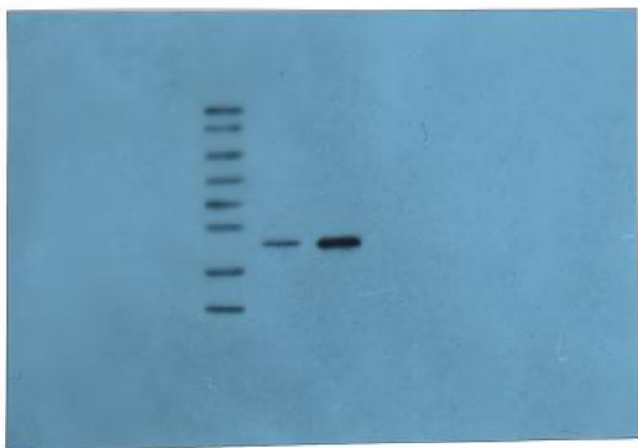
Fig 6F-1 FOSL1
