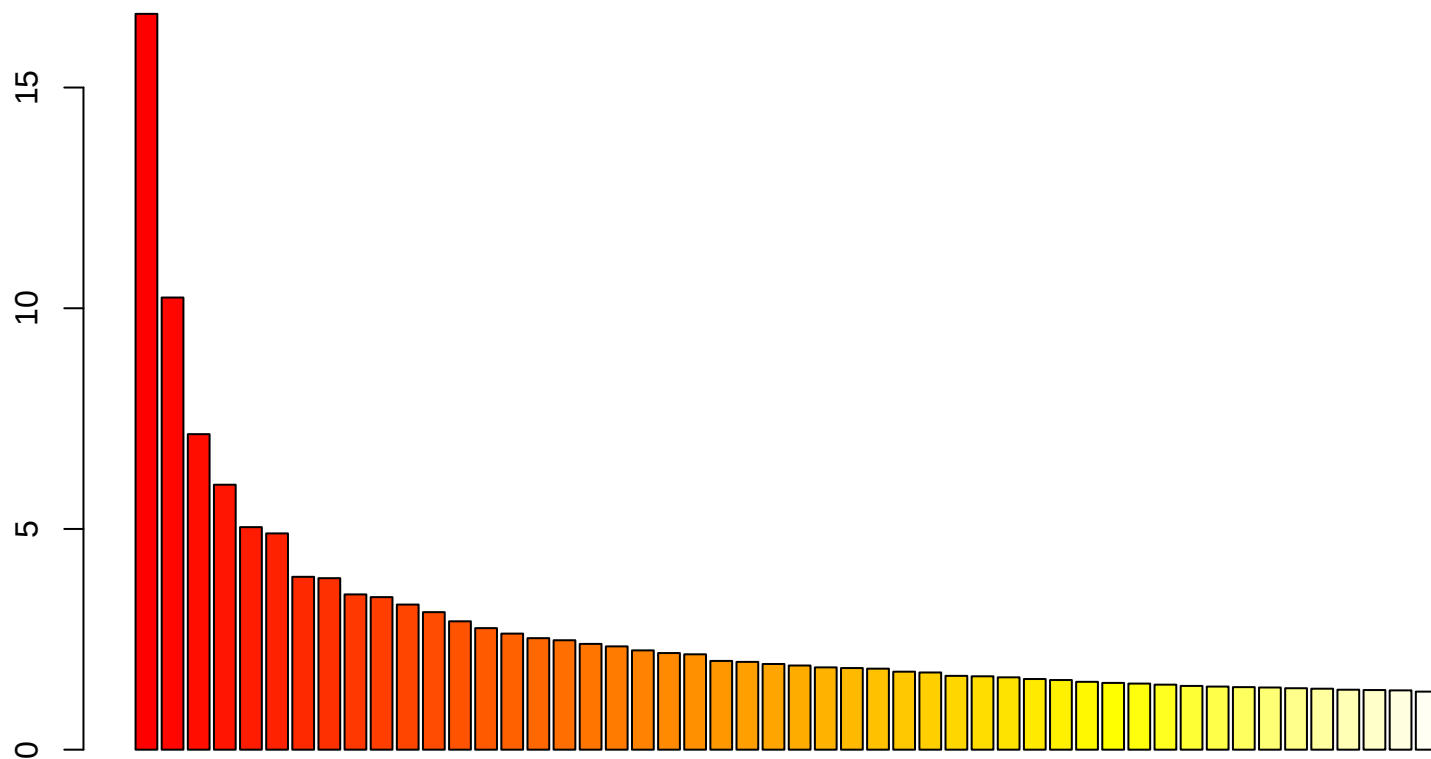
Hazelnut Diversity PCA eigenvalues
