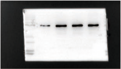
CPT1B
