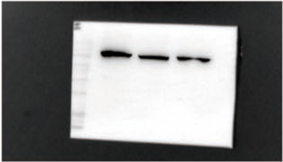
3E CPT1A
