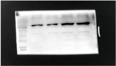
2E CPT1A
