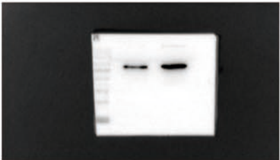
3B CPT1A
