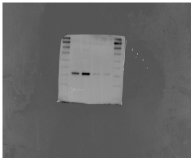
VEGF
