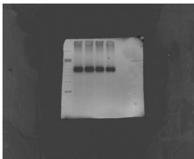
Tubulin
