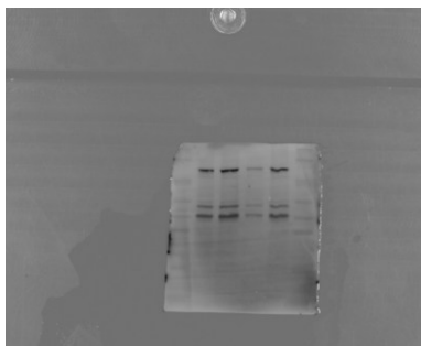
p-AKT
