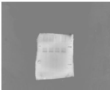
AKT
