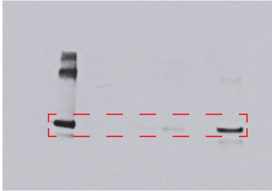
His-MBP-TRF1
