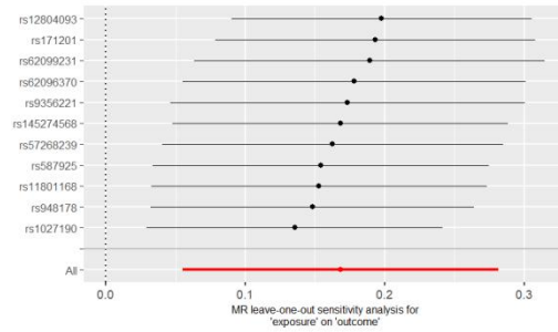
Depression(FinnGen) on CAD
