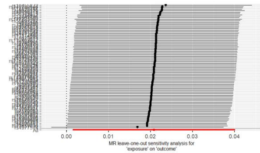
MI on Depression(FinnGen)
