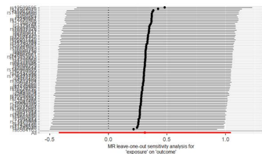
Depression(FinnGen) on MI
