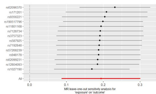
Depression(FinnGen) on Hypertension
