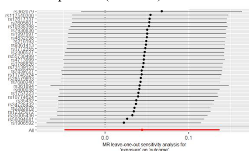
HF on Depression(FinnGen)
