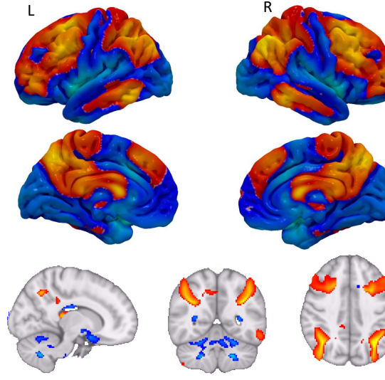
ANM using parahippocampal tau
