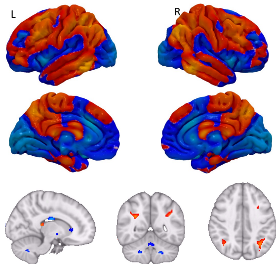
ANM using entorhinal tau
