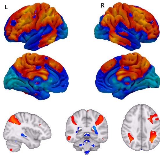
ANM using amygdala tau
