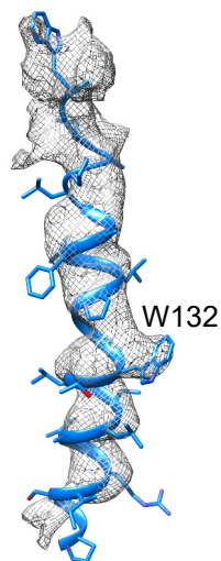
TM4
