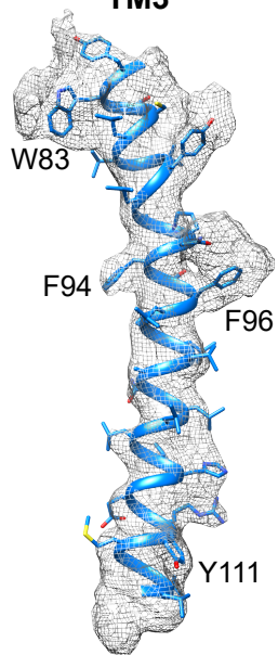
TM3
