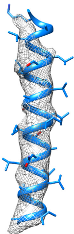
TM1
