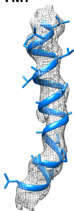
TM7
