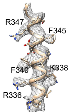
G \alpha 4
