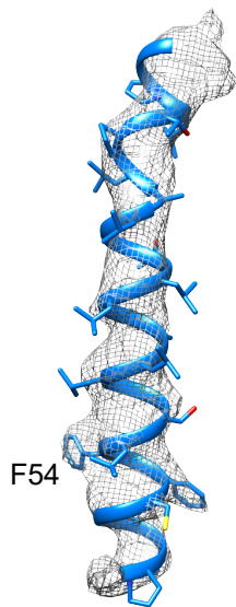
TM2
