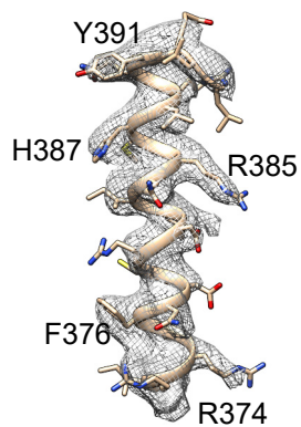
G \alpha 5
