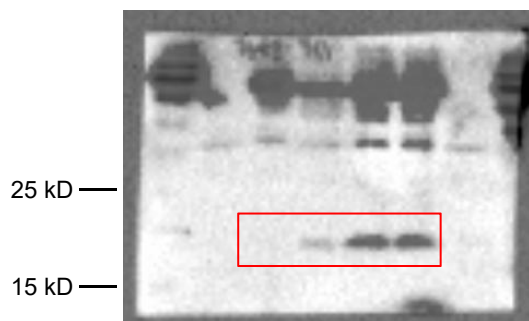
IL-18
