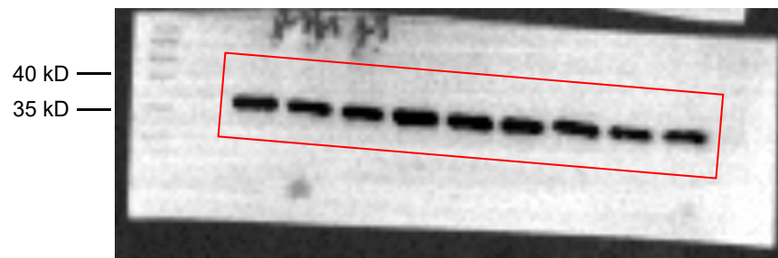
Pro-IL-1 \beta
