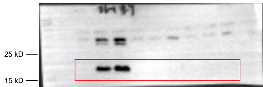
IL-1 \beta
