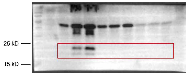
p20
