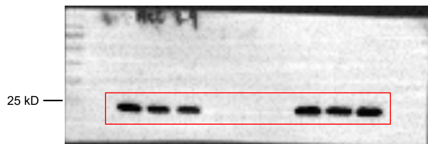
ASC
