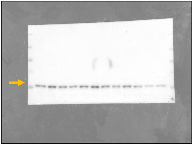
Smad7 (50 KDa)
