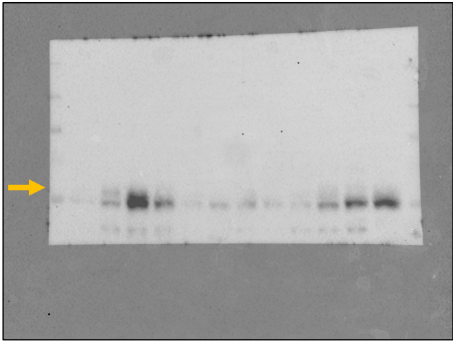
Smad4 (60 KDa)
