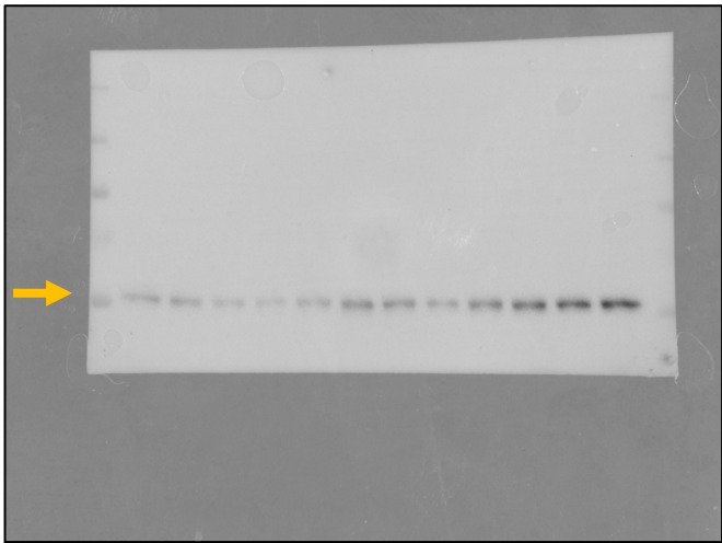
Smad3 (48 KDa)
