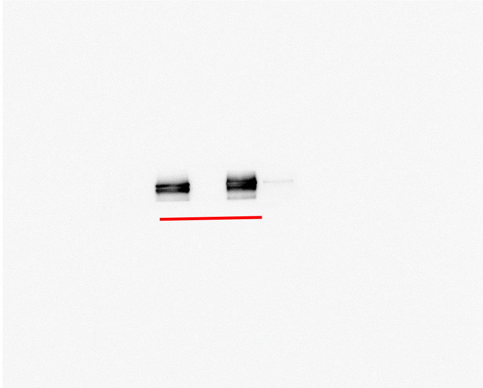
Fig 4B DHX9
