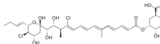
enacyloxin
