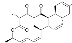
anthracimycin
