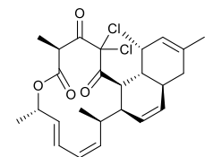
chlorotonil
