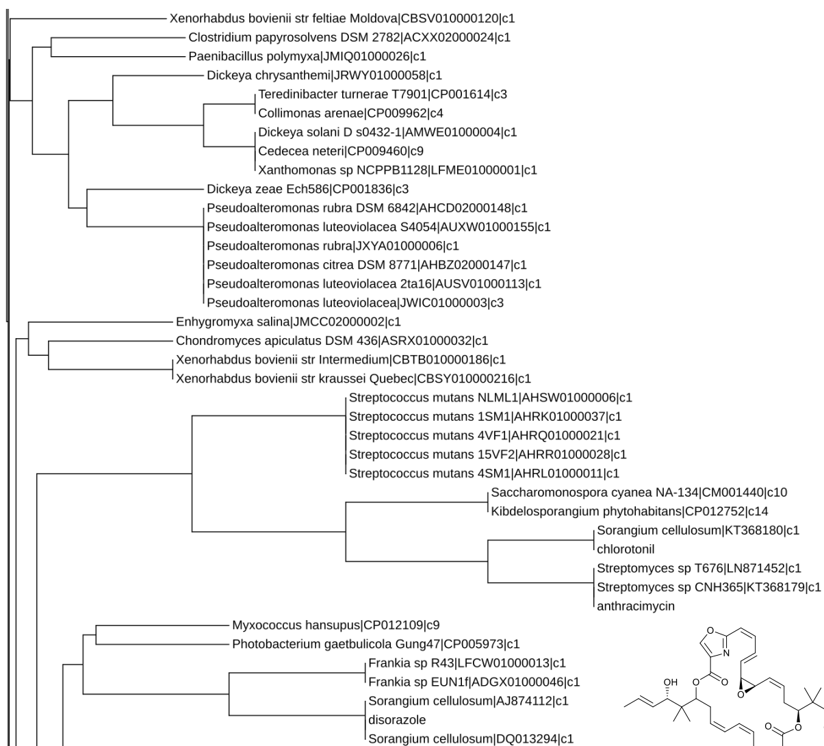
chlorotonil
