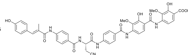
albicidin
