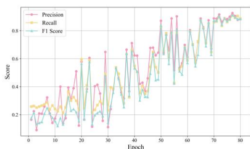
InceptionNeXt-Validation
