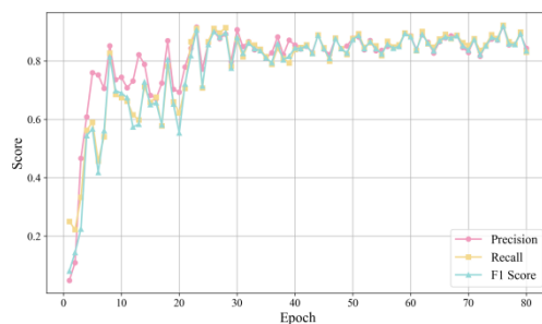
GhostNetV3-Validation
