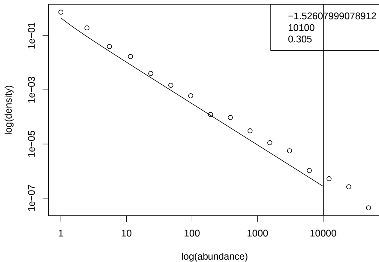
TARA_030.SUR.180.2000.DNA
