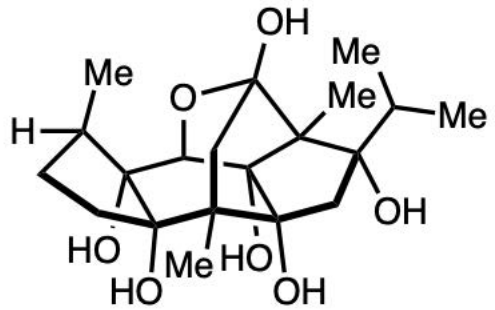
(+)-perseanol (3)
