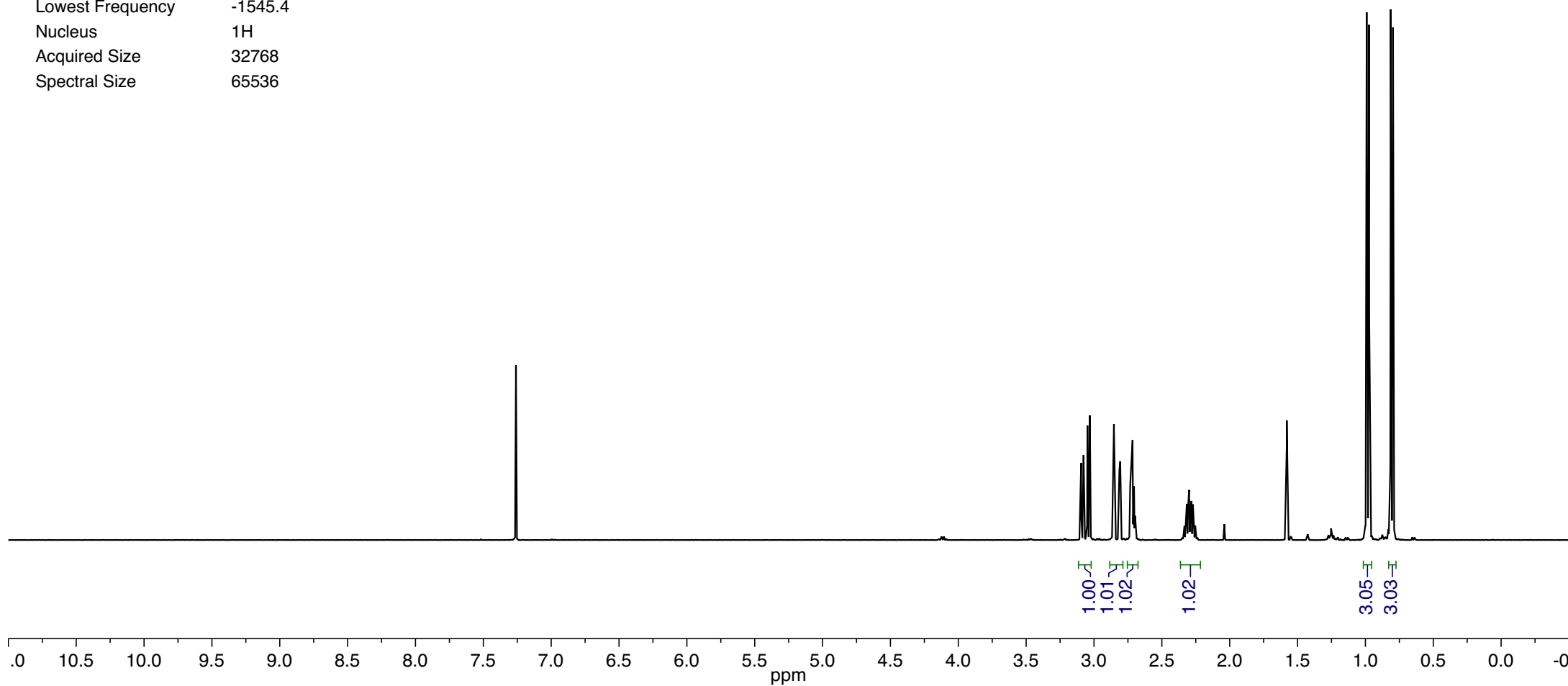
(±)-24
