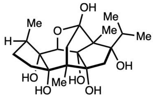
(+)-perseanol (3)
