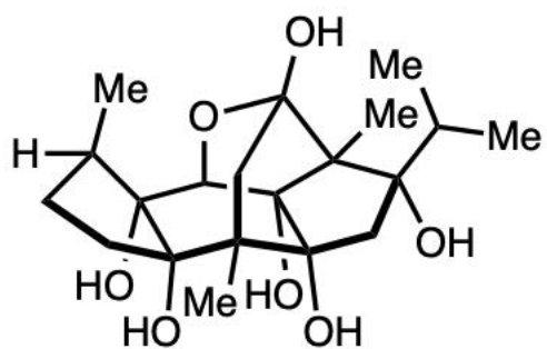
(+)-perseanol (3)
