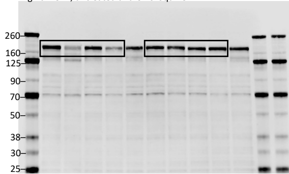
Fig 4c. EGFR, M6P
