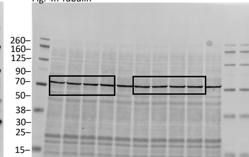
Fig. 4n Tubulin
