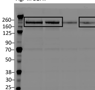
Fig. 4h EGFR
