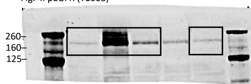
Fig. 4i pAKT
