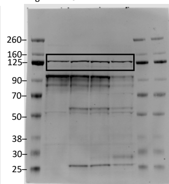
Fig. 4k VINC
