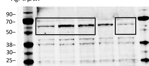
Fig. 4i pAKT
