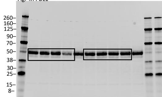
Fig. 4n PDL1
