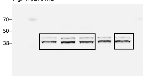
Fig. 4i pERK1/2
