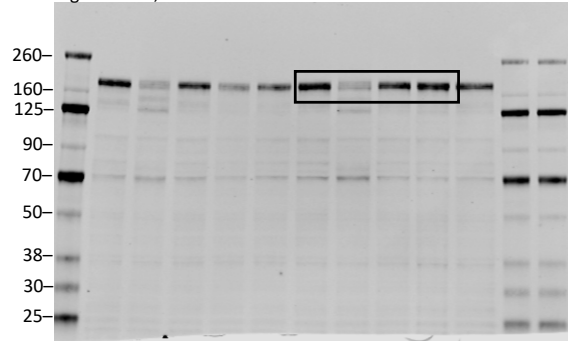
Fig 4d. EGFR
