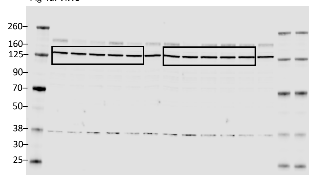
Fig 4d. VINC
