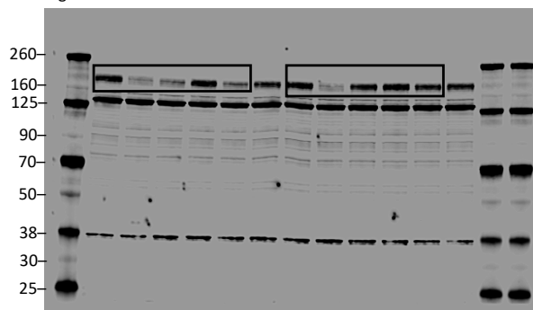
Fig 4d. EGFR
