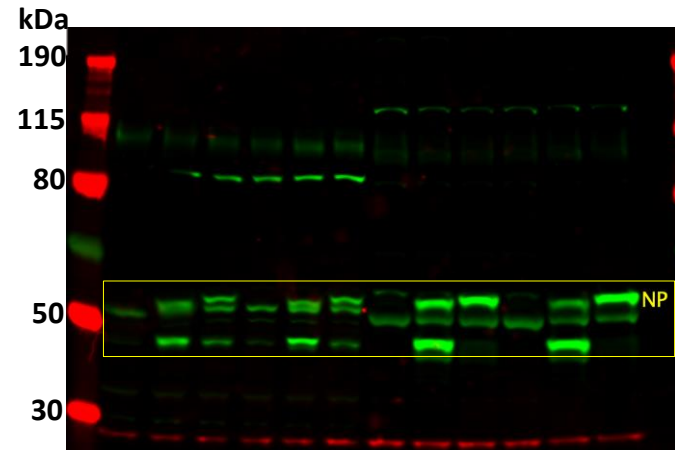
Gel run using MES buffer
