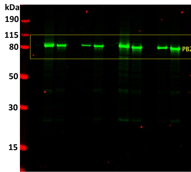
Gel run using MES buffer
