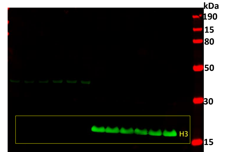
Gel run using MES buffer
