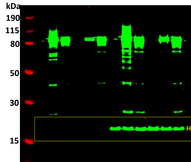
Gel run using MES buffer
