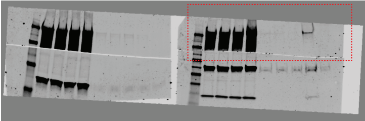
PxP RPB1
