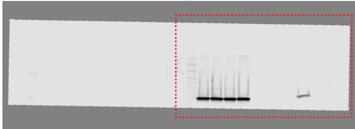
Input H3
