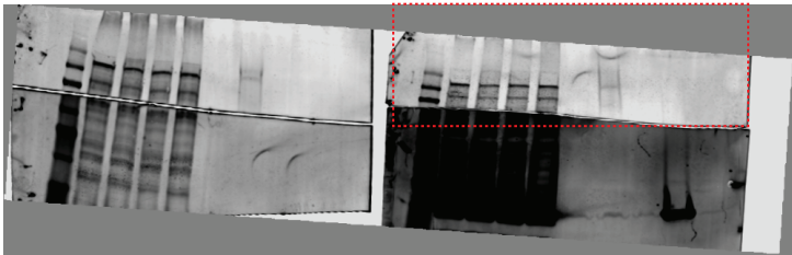
PxP DNMT1
