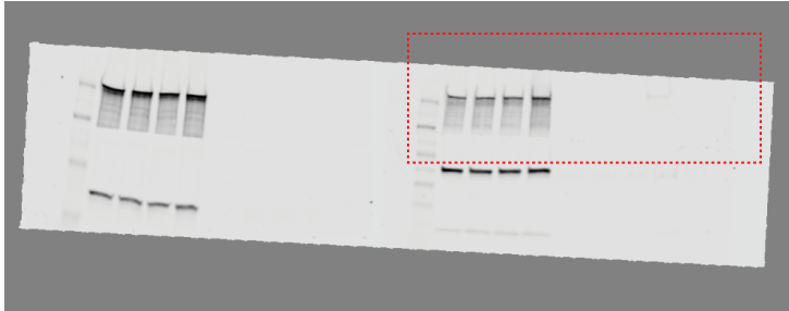
Input RPB1
