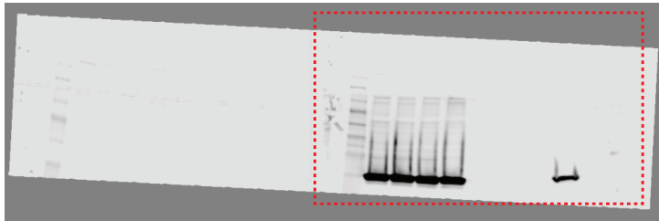
PxP H3
