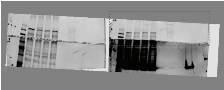
Input DNMT1
