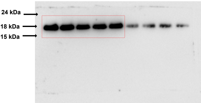
H3K36me3
