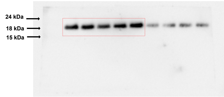
H3K9me3
