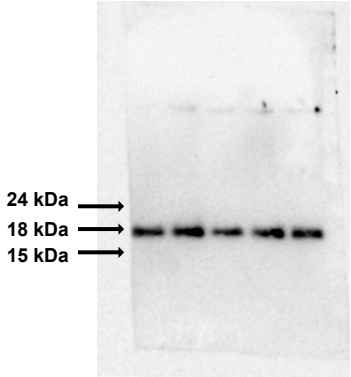
H3K36me3
