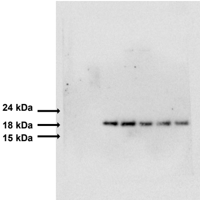
H3K4me3
