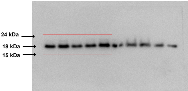
H3K79me3
