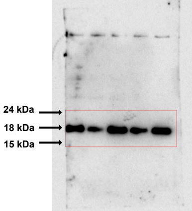
H3K36me3
