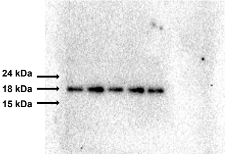
H3K27me3
