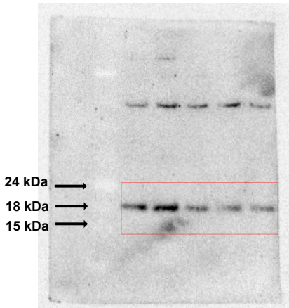
H3K79me3
