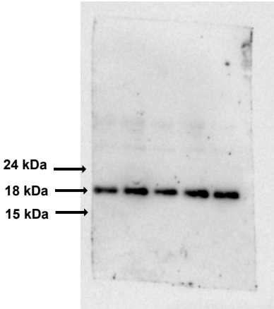
H3K27me3
