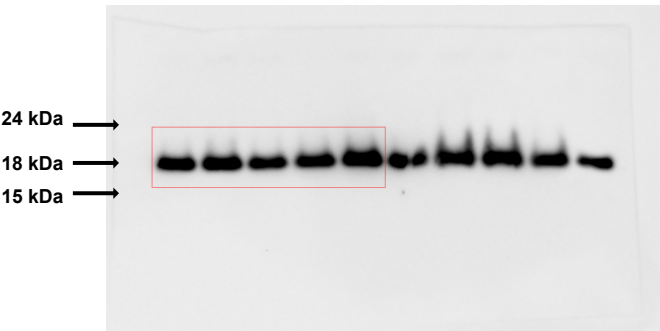
H3K27me3
