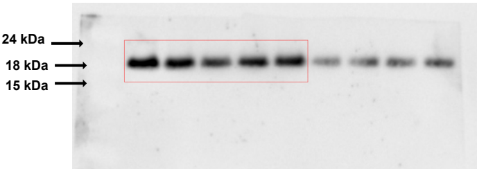
H3K4me3
