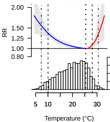
Uruguaiana, Brasil Mean temp. 19.9C
