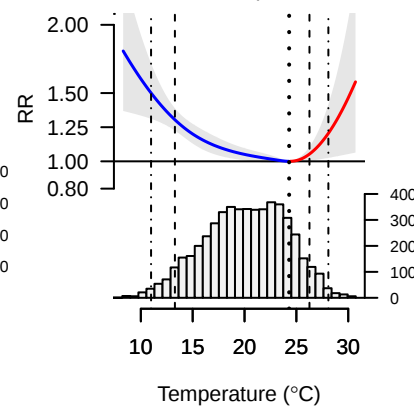
Tubarão, Brasil Mean temp. 20C
