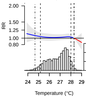
São Luís, Brasil Mean temp. 26.7C
