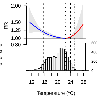
Varginha, Brasil Mean temp. 19.9C
