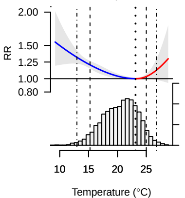
Taubaté, Brasil Mean temp. 20.4C
