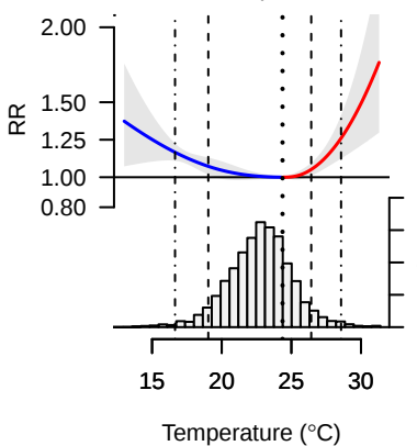
Uberaba, Brasil Mean temp. 22.7C
