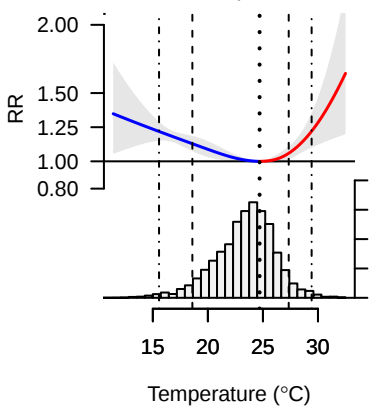
São José do Rio Preto, Brasil Mean temp. 23.3C
