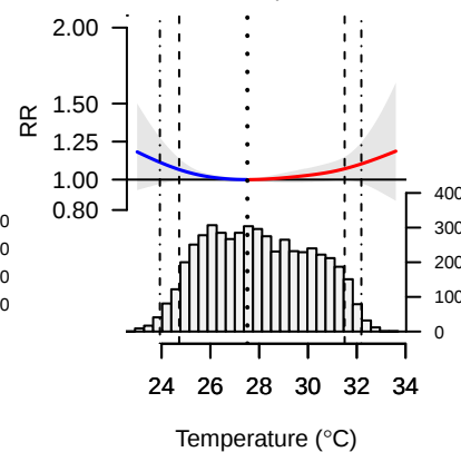
Teresina, Brasil Mean temp. 27.8C
