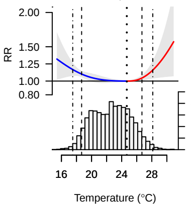
Teófilo Otoni, Brasil Mean temp. 22.6C
