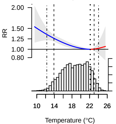
Teresópolis, Brasil Mean temp. 18.7C
