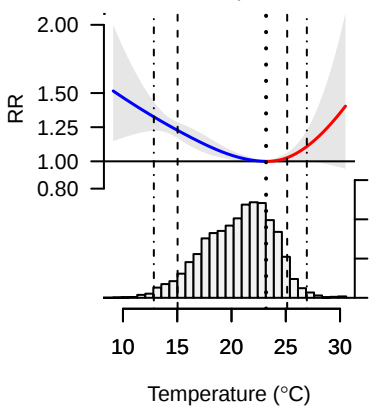
Tatuí, Brasil Mean temp. 20.5C
