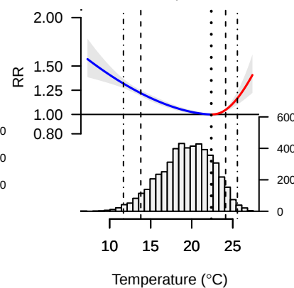
São Paulo, Brasil Mean temp. 19.3C
