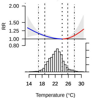
Uberlândia, Brasil Mean temp. 22.2C
