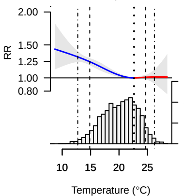
São José dos Campos, Brasil Mean temp. 20.1C
