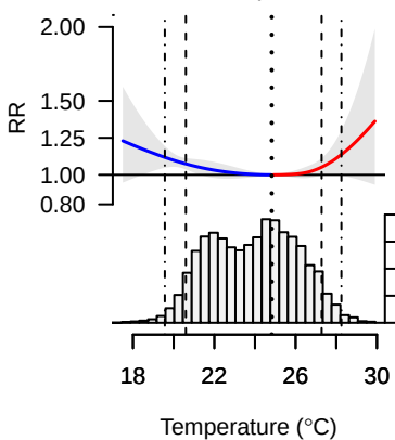
Teixeira de Freitas, Brasil Mean temp. 23.9C
