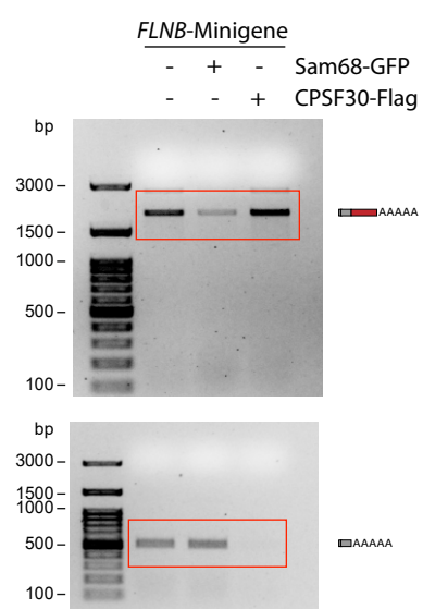
Fig. 6i RT-PCR
