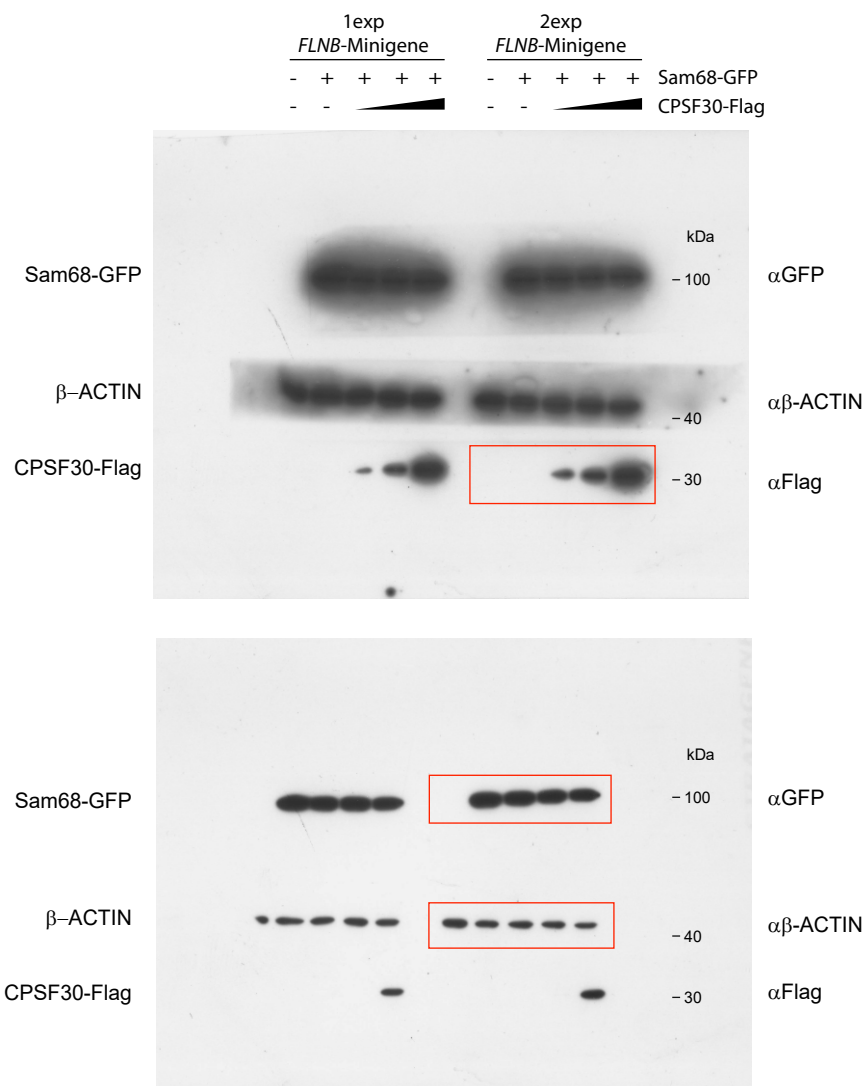
Fig. 6j Western-blot
