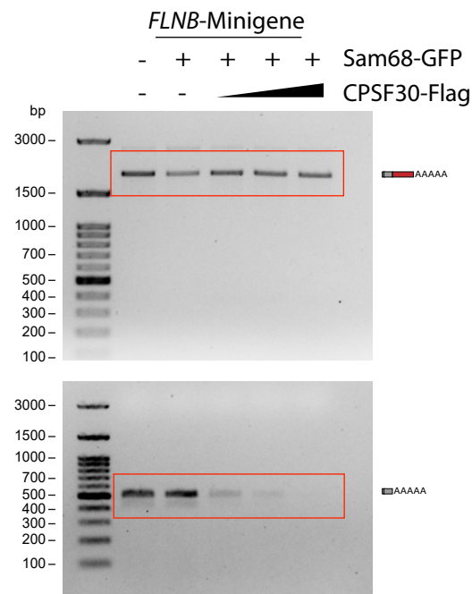
Fig. 6j RT-PCR
