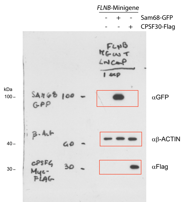
Fig. 6i Western-blot
