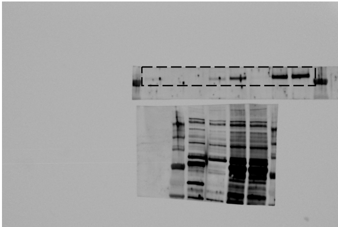
Anti-Pol eta
