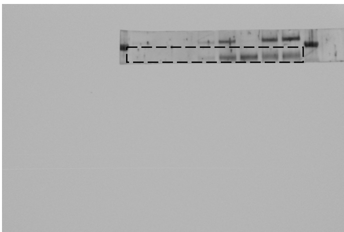
Anti-Pol eta
