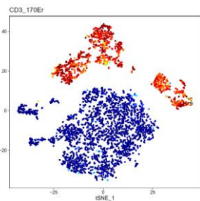
CD3_170Er
