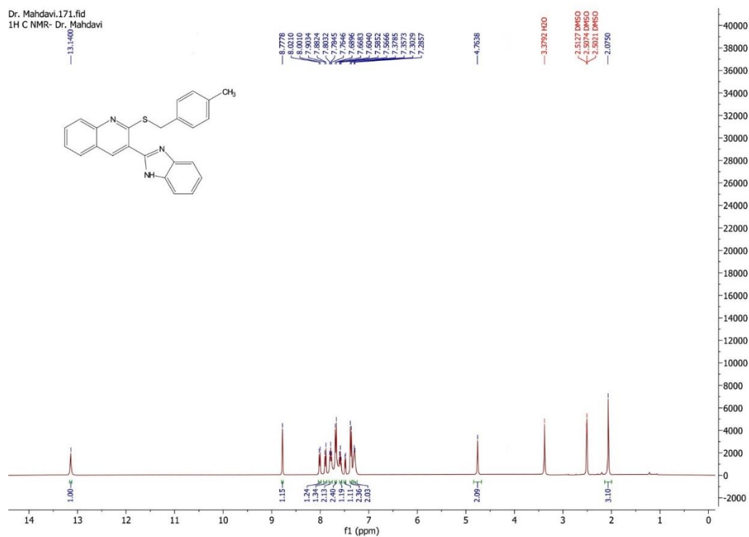
Fig. S14. 3-(1H-benzo[d]imidazol-2-yl)-2-((4-methylbenzyl)thio)quinolone ( 6n )
