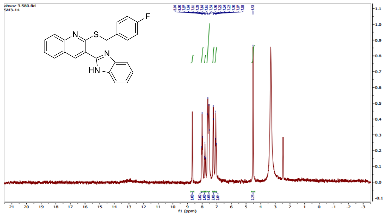
Fig. S4. 3-(1H-benzo[d]imidazol-2-yl)-2-((4-fluorobenzyl)thio)quinolone ( 6d )
