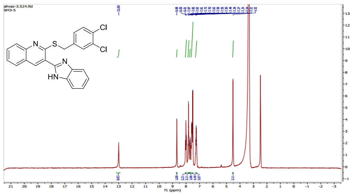
Fig. S11. 3-(1H-benzo[d]imidazol-2-yl)-2-((3,4-dichlorobenzyl)thio)quinolone ( 6k )
