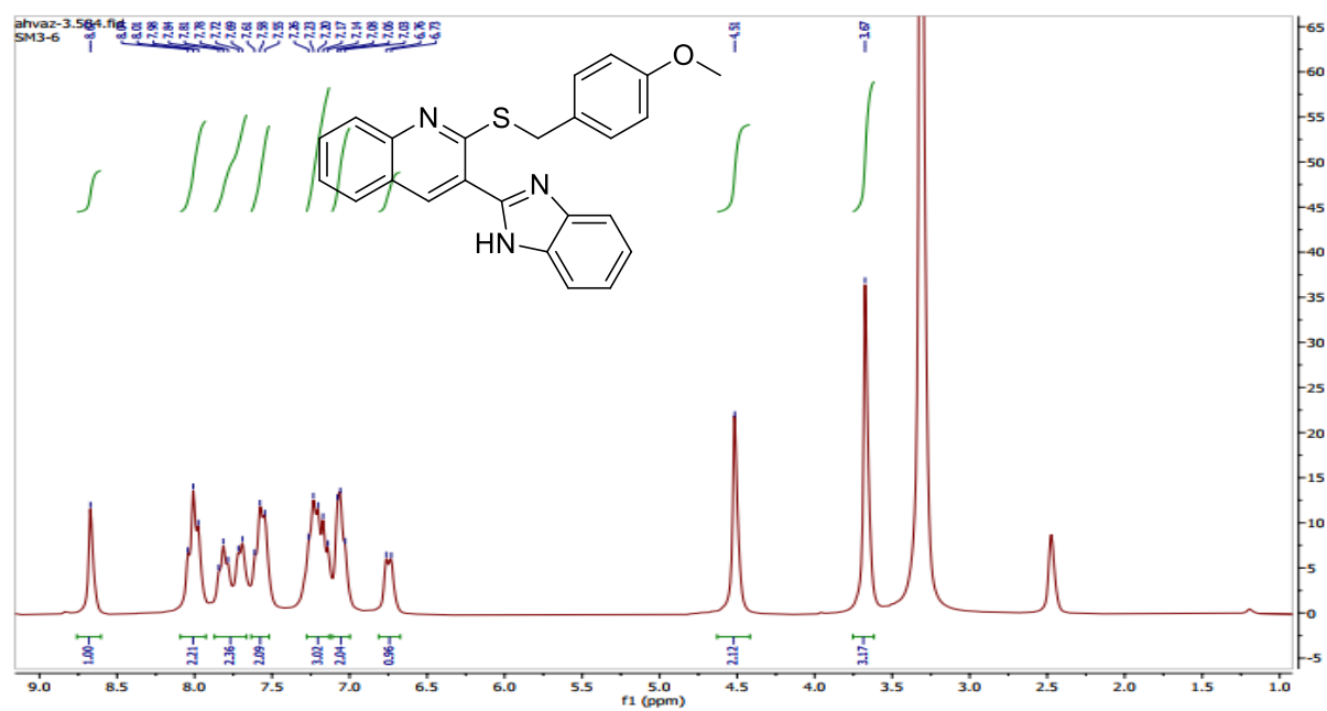
Fig. S17. 3-(1H-benzo[d]imidazol-2-yl)-2-((4-methoxybenzyl)thio)quinolone ( 6q )
