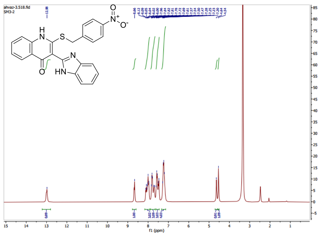
Fig. S16. 3-(1H-benzo[d]imidazol-2-yl)-2-((4-nitrobenzyl)thio)quinolone ( 6p )
