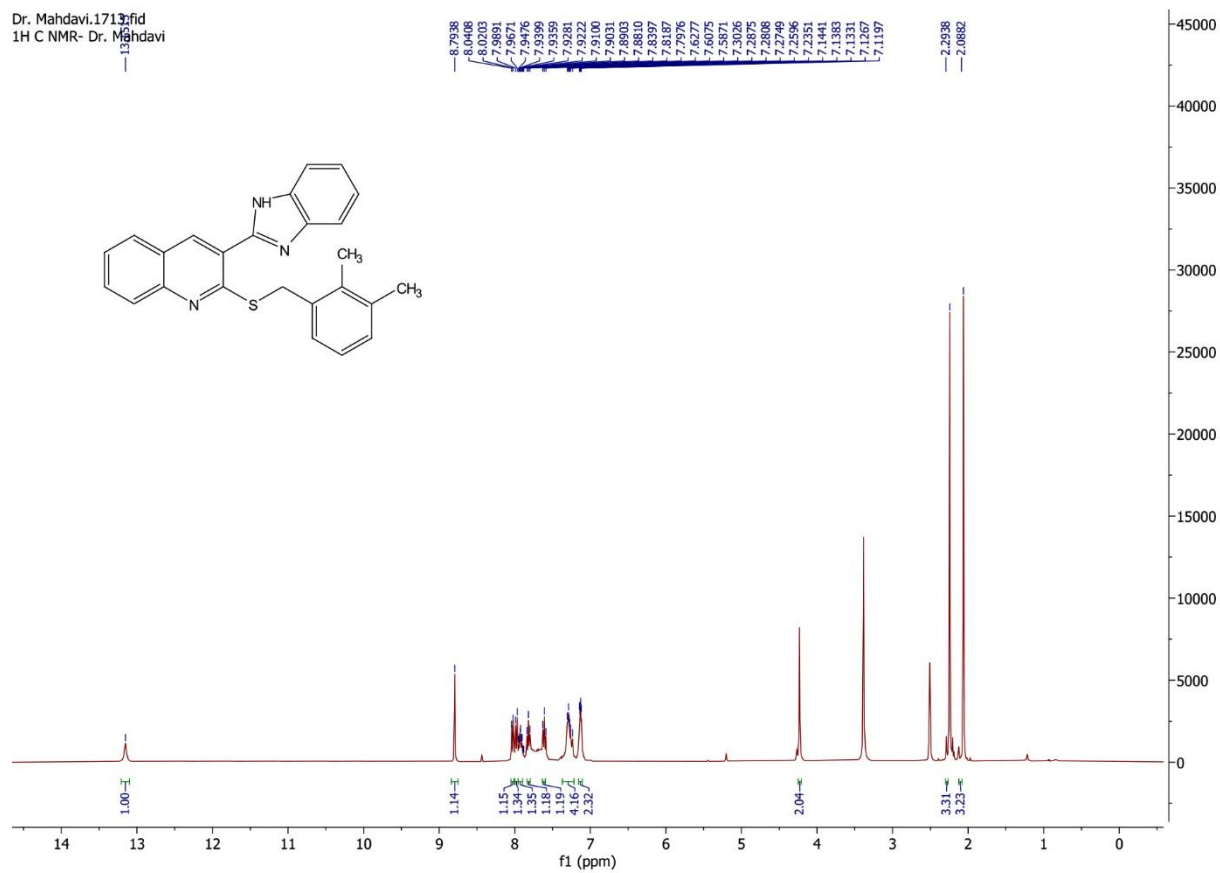
Fig. S15. 3-(1H-benzo[d]imidazol-2-yl)-2-((2,3dimethylbenzyl)thio)quinolone ( 6o )
