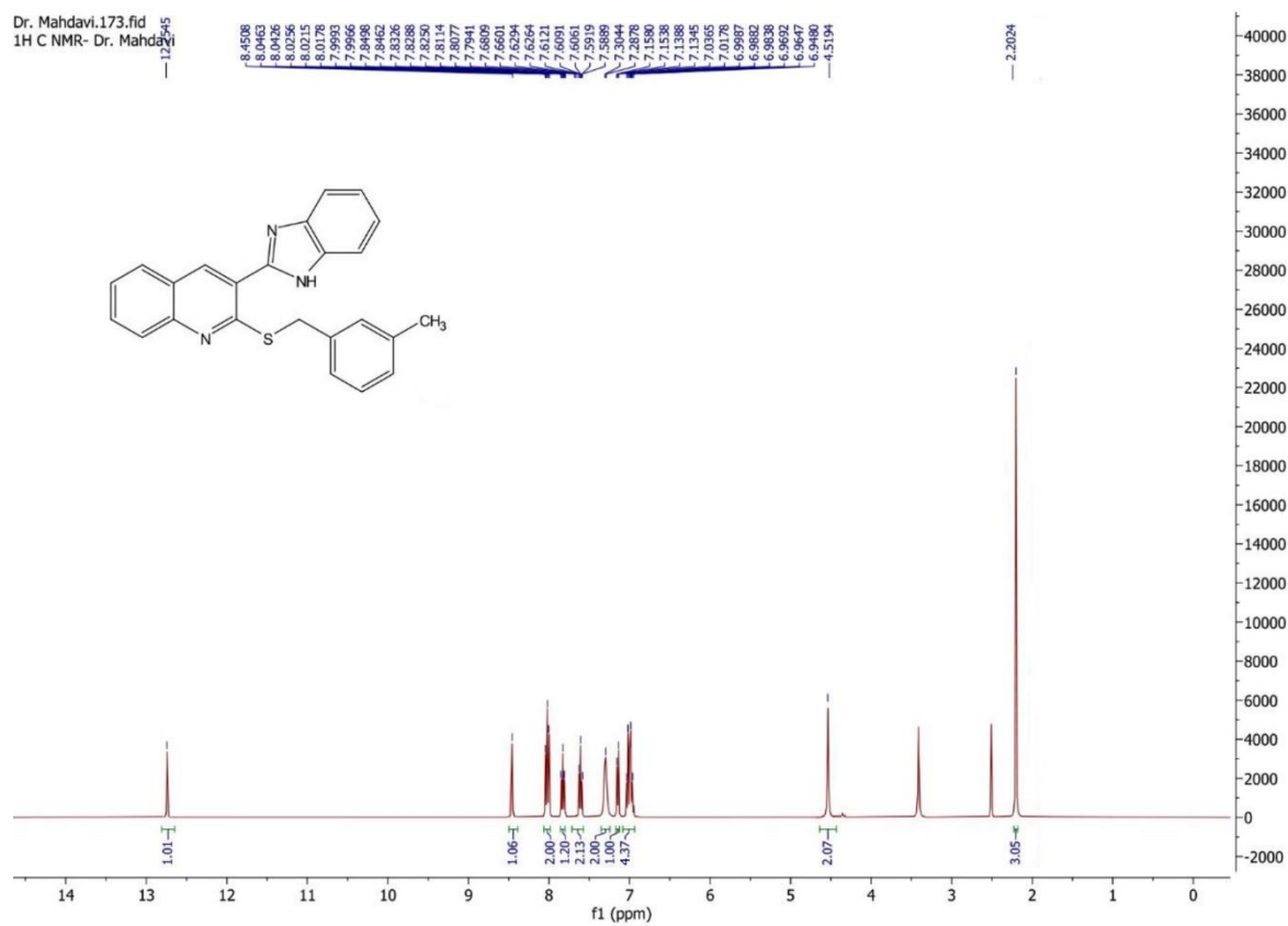
Fig.S13.3-(1H-benzo[d]imidazol-2-yl)2-((3-methylbenzyl)thio)quinolone(6m)
