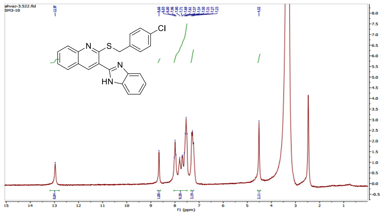
Fig. S7. 3-(1H-benzo[d]imidazol-2-yl)-2-((4-chlorobenzyl)thio)quinolone ( 6g )
