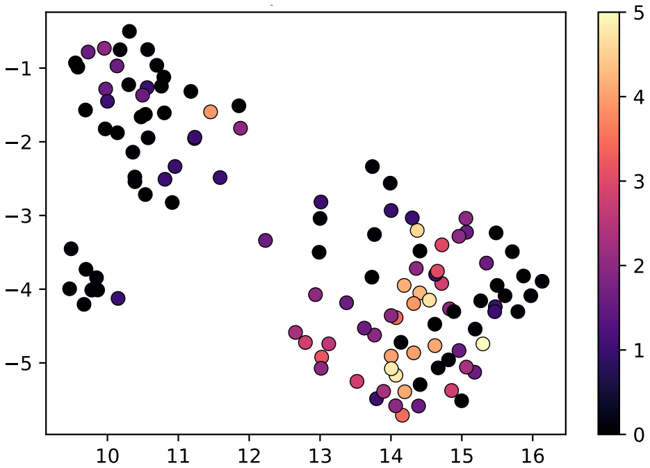
ago2-1 (Smp_179320)
