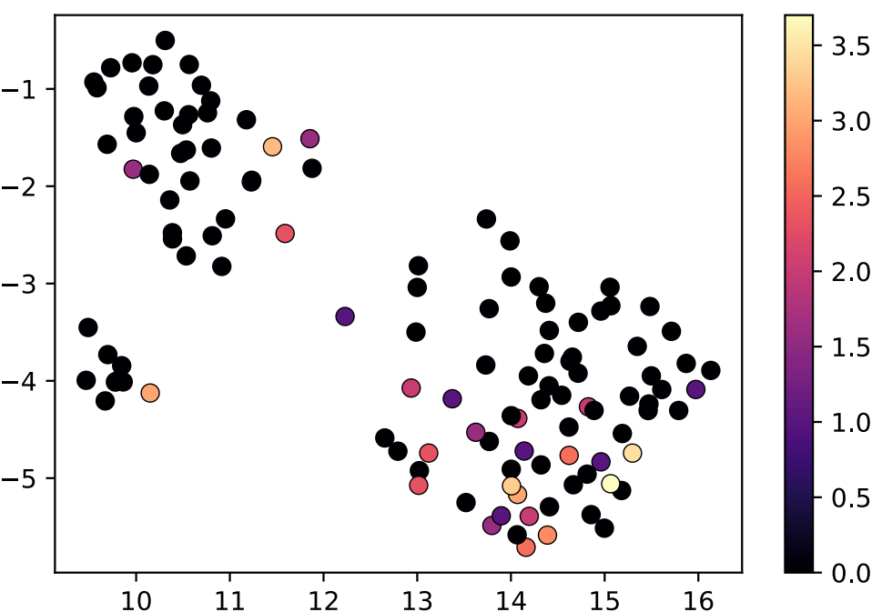
Zfp-1 (Smp_145470)
