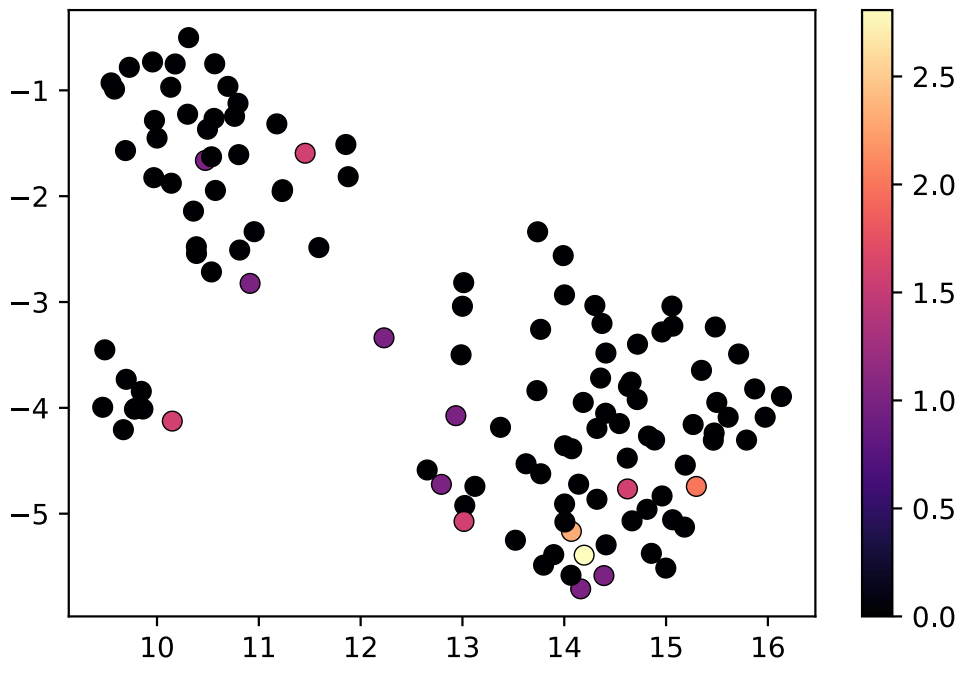
fgfrA (Smp_175590)
