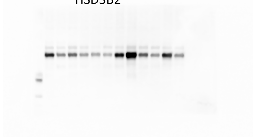
HSD3B2
