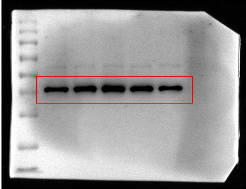
Fig. 9A \beta -actin
