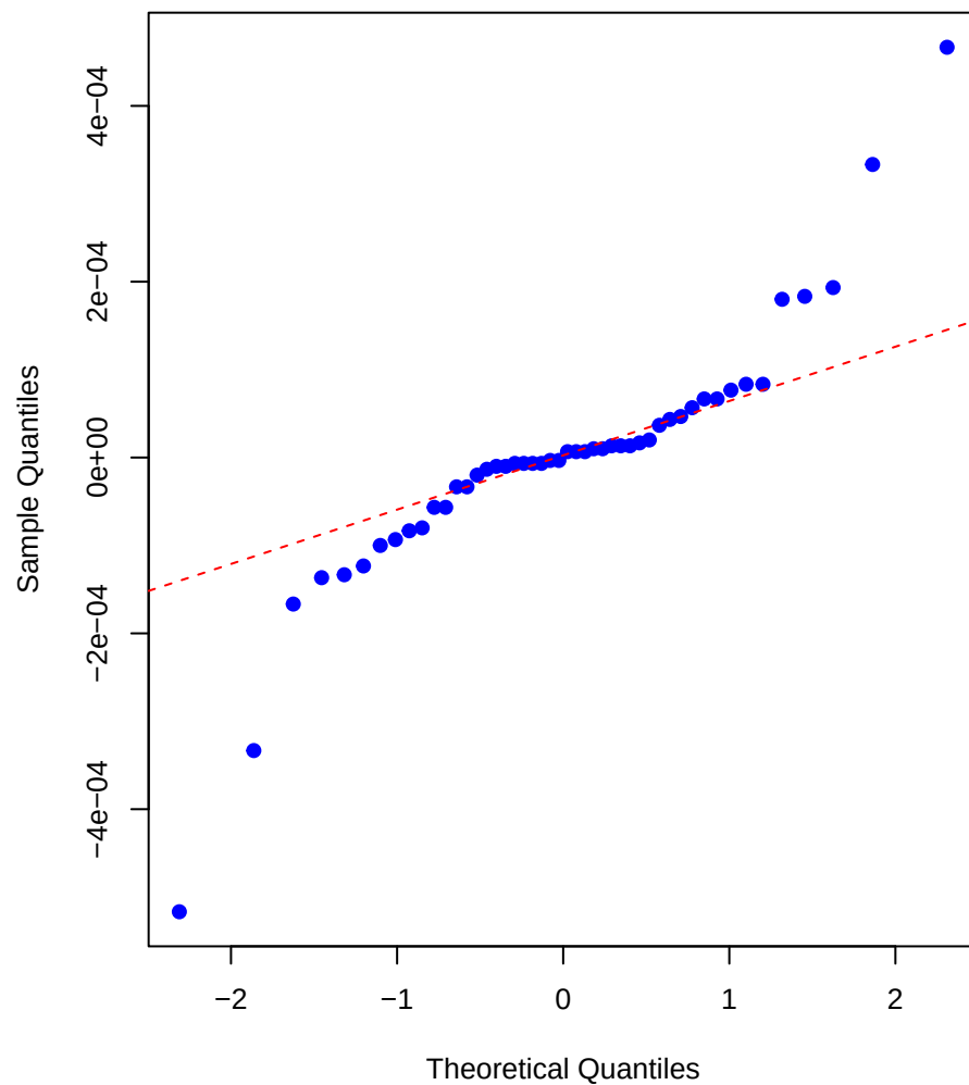
Zinc (Zn) – Q-Q Plot
