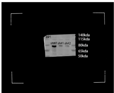
Fig3B-F13A1
