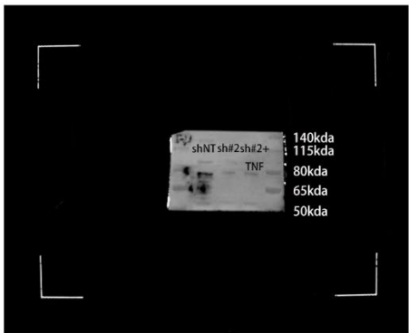
Fig6A-IKK \alpha
