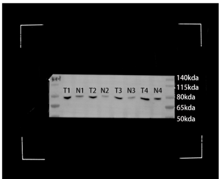
Fig2L-F13A1
