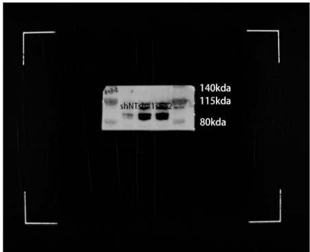
Fig6A-F13A1
