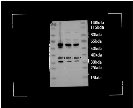
Fig5E-Vimentin
