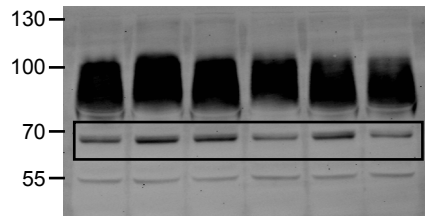
anti-S6K
