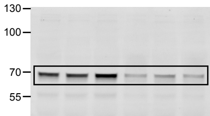
anti-pS6K
