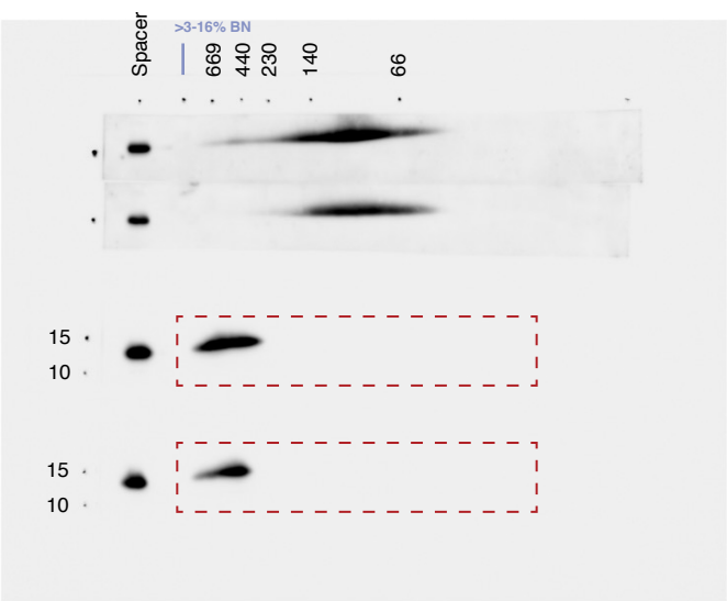
CI: NDUFB6
