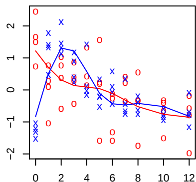
ZK1058.6
