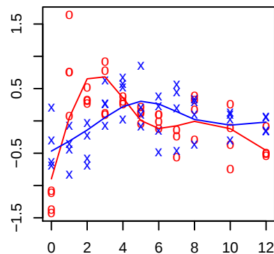
F56F3.2
