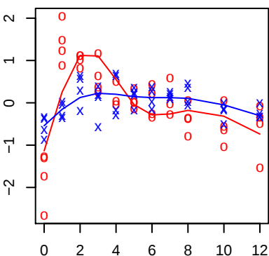
Y53F4B.C
