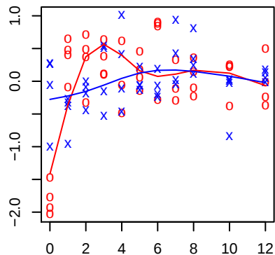
K09C4.8
