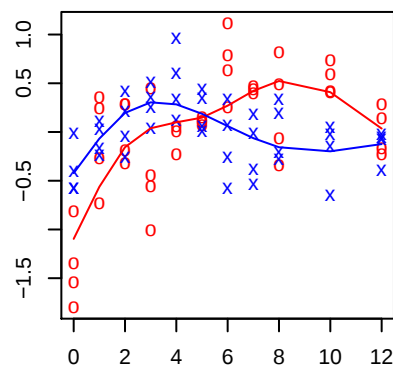
F56H11.6
