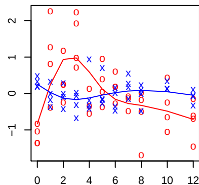
Y45F10D.2
