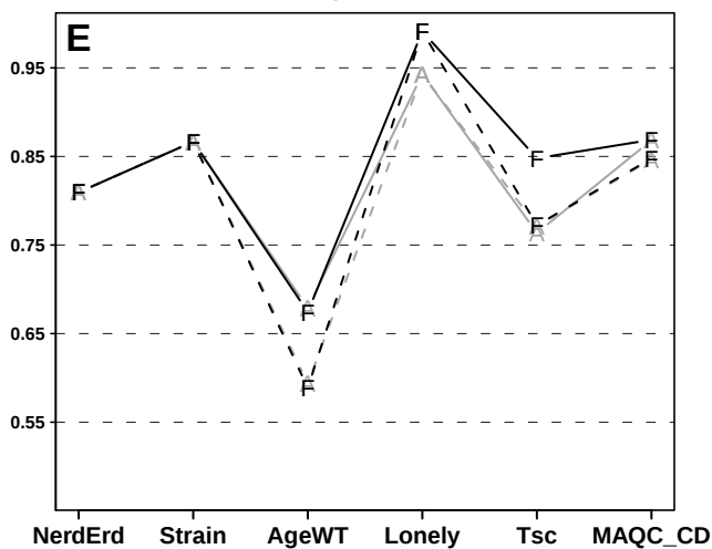
t-test, GC-RMA
