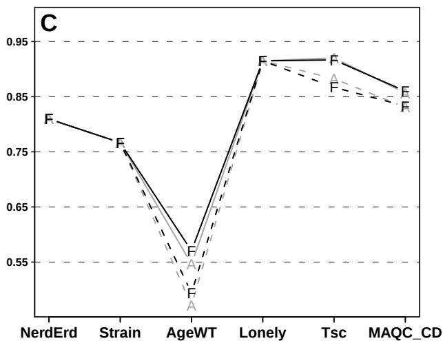
t-test, MBEImm
