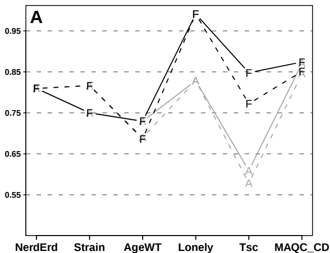
t-test, PLIER
