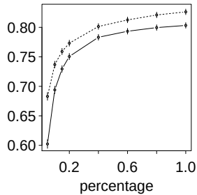
(d) AUC-PR
