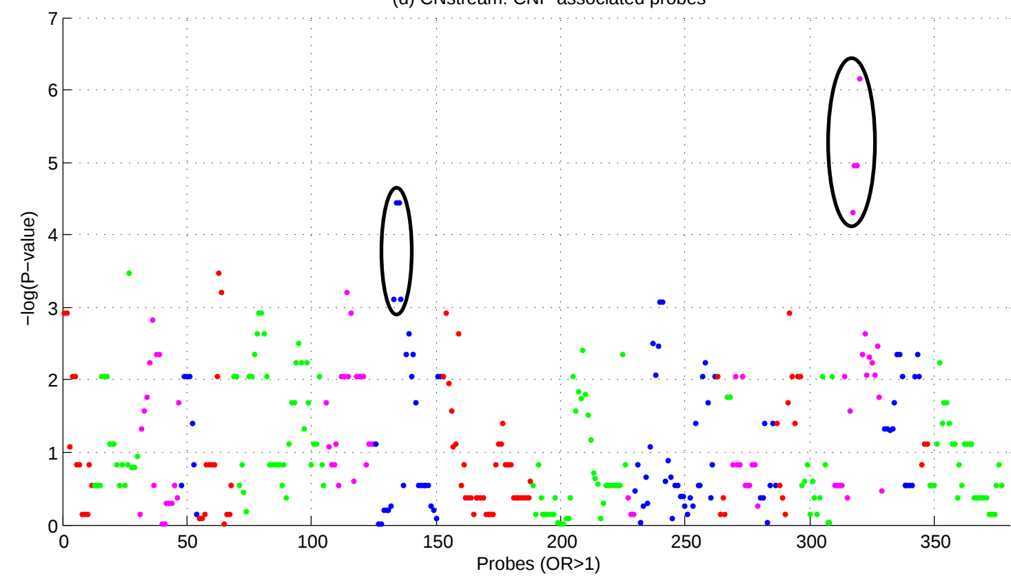
(d) CNstream: CNP associated probes
