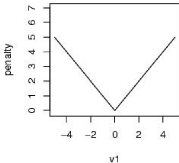
HL penalty with w=2 (LASSO)
