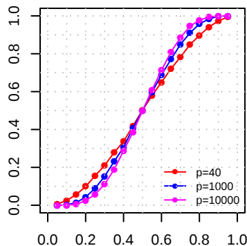
3-NN
