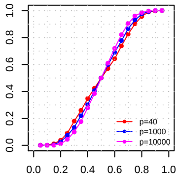
SVM
