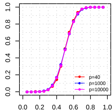
PLR
