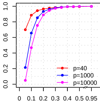
3-NN
