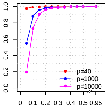
SVM
