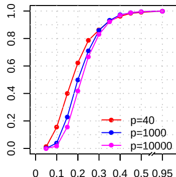
PLR
