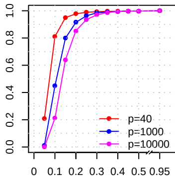
SVM
