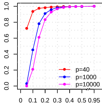
PLR
