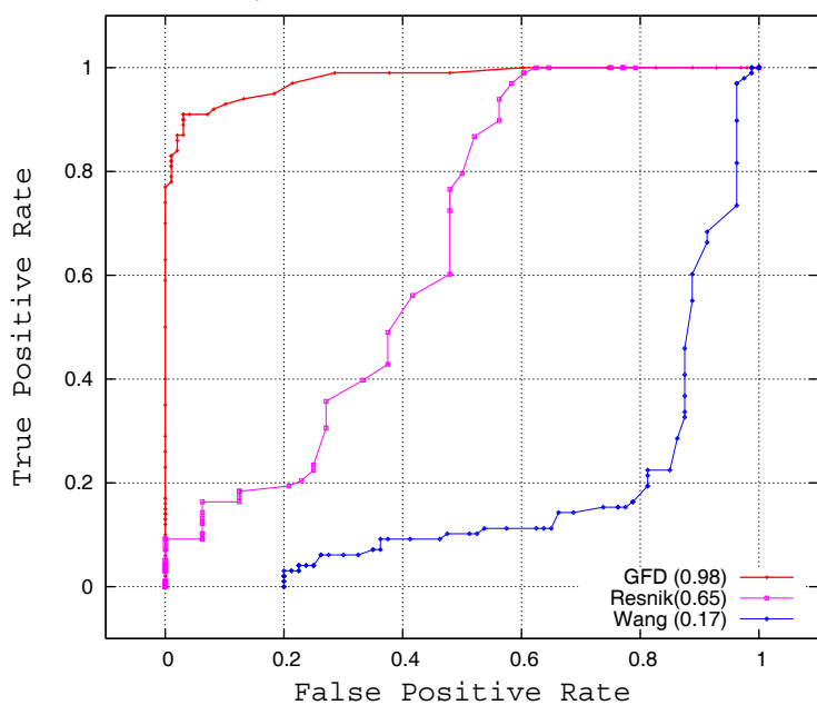
B) Molecular Function
