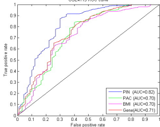
GSE4115 ROC curve
