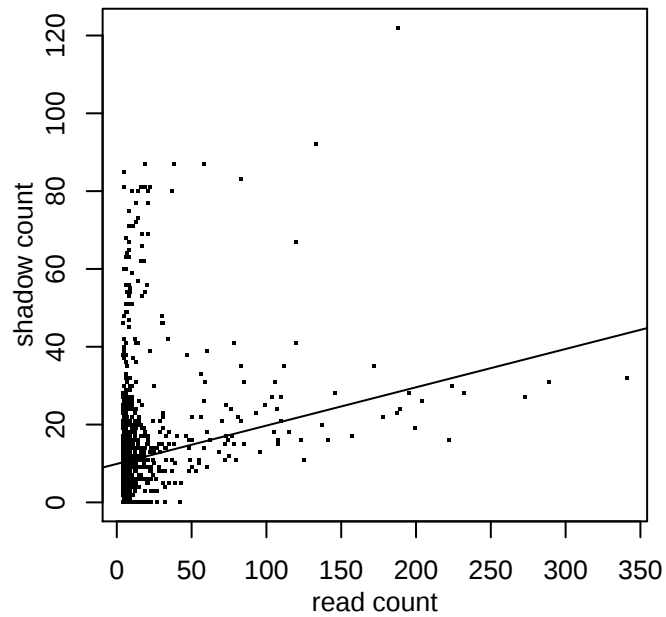
SAGE
