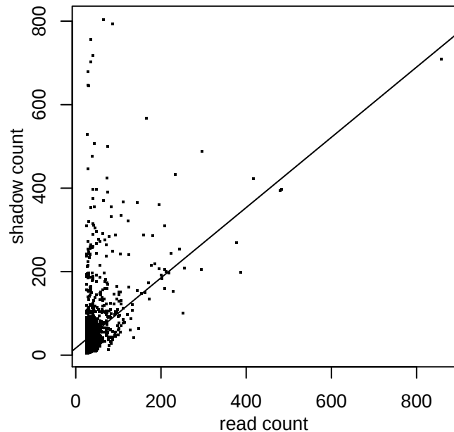
SAGE
