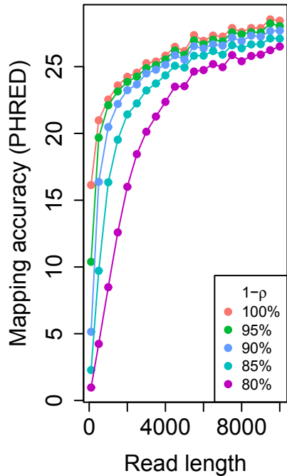
H. sapiens
