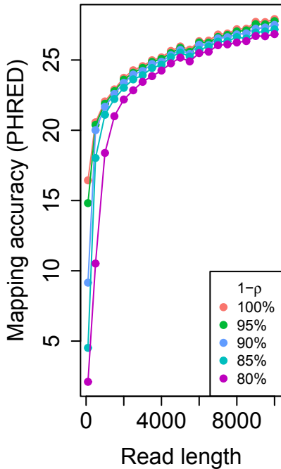
A. thaliana
