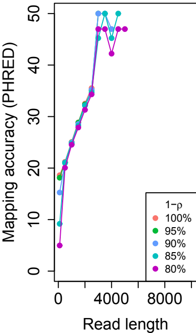
E. coli
