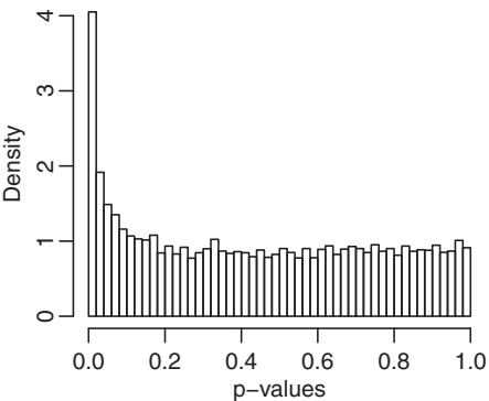
Separate
