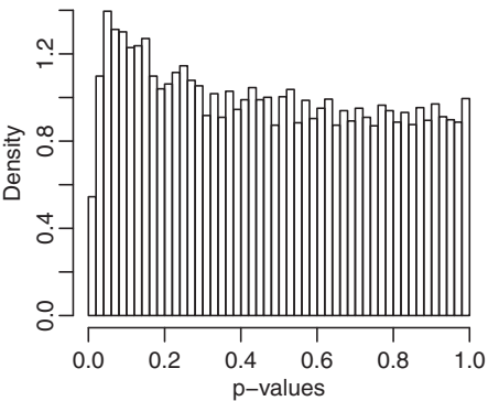
maanova
