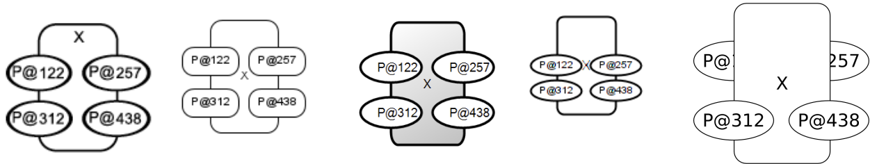
neuronal_muscle_signalling.abgn
