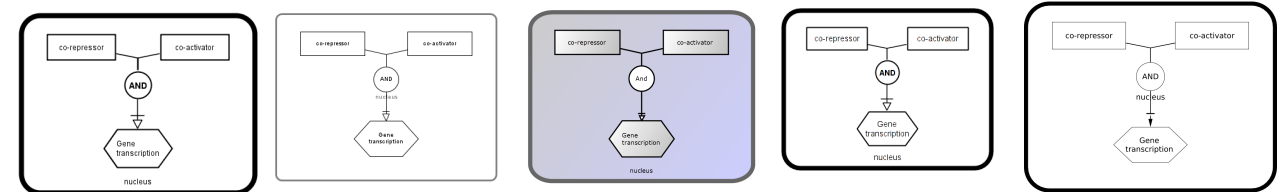
delay.sbgm
