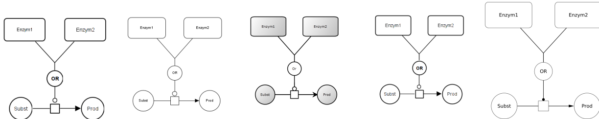
bool-cxpr.pd.sbgm
