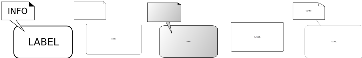
reversible-vertical.pn.sbgm
