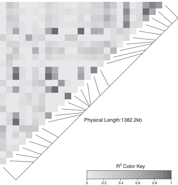
Pairwise LD
