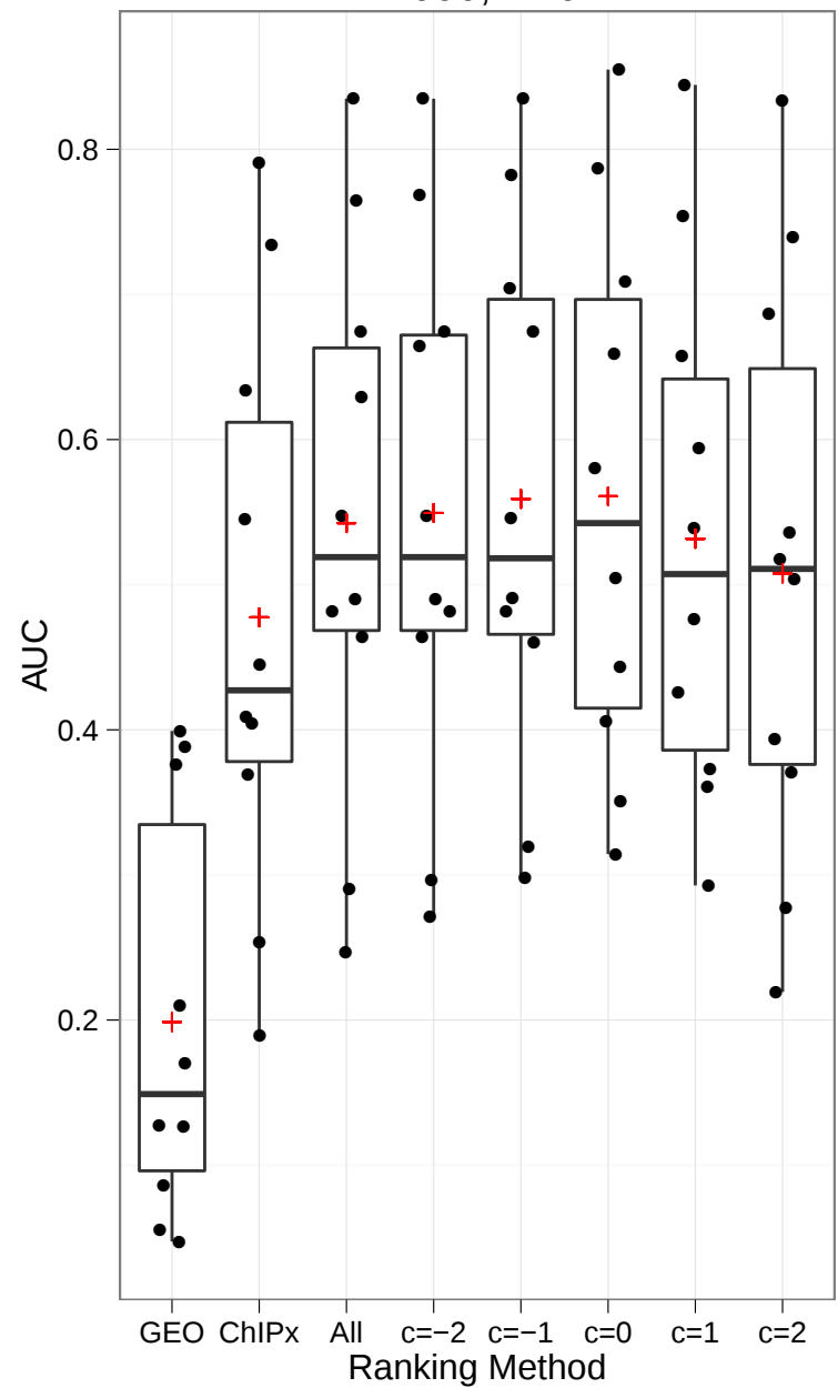
n=1000, w=0.1
