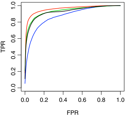
ROC
